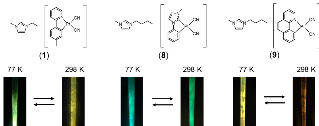
図 3. 白金(II)錯体イオン液体の分子構造と発光写真の温度変化
