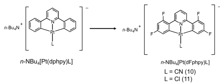
図 4. 三座配位子に対するフッ素導入による分子設計
