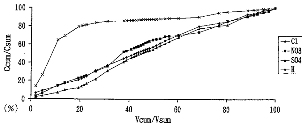
図-1 春期融雪水中における融雪水量と \text{H}^+ およびアニオンの溶出量との関係 ( C_{\text{sum}} :全溶出成分量、 C_{\text{cum}} :積算溶出成分量、 V_{\text{sum}} :全流出水量、 V_{\text{cum}} :積算溶出水量)
