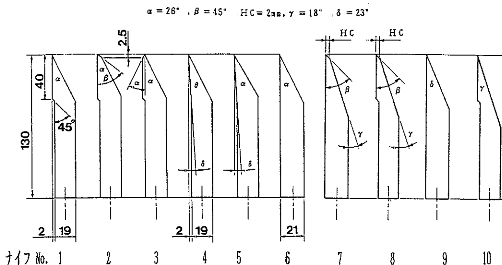
図-1 ナイフ別刃先断面図
