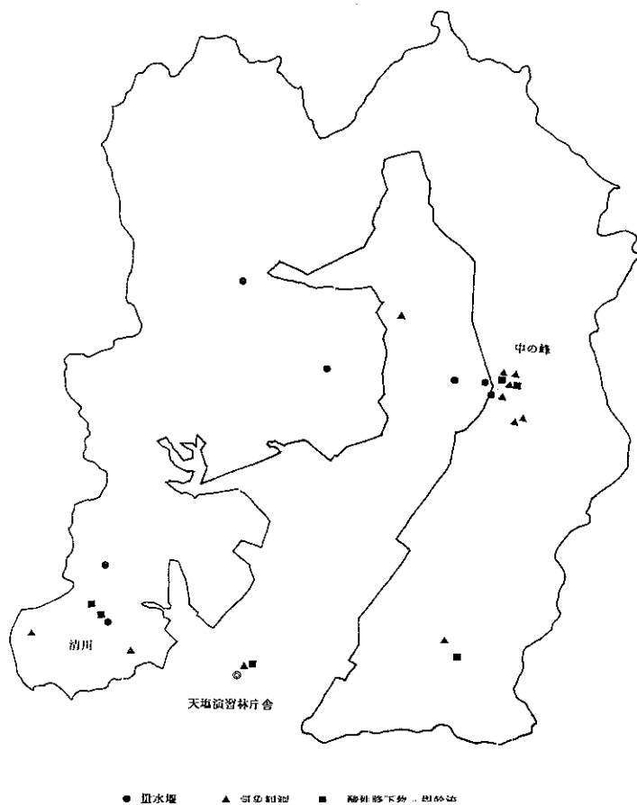
図-2 1995年度の流域観測設備
