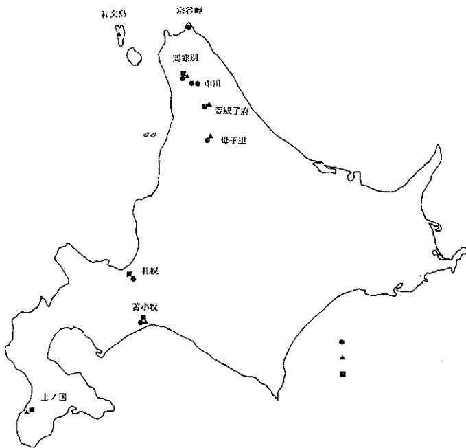
図－4 北大演習林の流域観測設備（他に和歌山演習林で流量観測）
