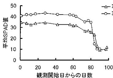
図-4 葉緑素計によるミズナラ (2 個体) の観測開始日からの日数と平均SPAD値
