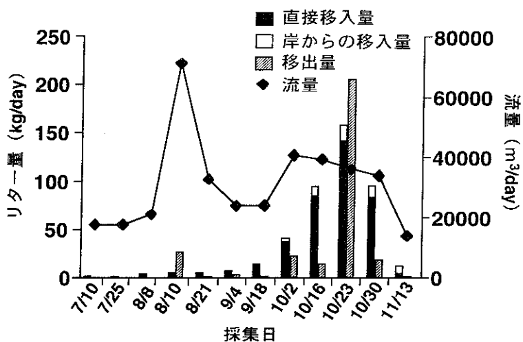
図-2 幌内川におけるリター移流量と河川水流量の季節変動
