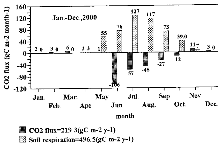
図-4 土壌呼吸量とCO2フラックスの季節変化、2000年
