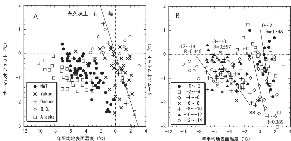
図7：北米におけるサーマルオフセットと年平均地表面温度との関係。
