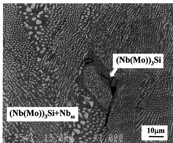
Fig. 4 BEI micrograph of Nb–19Si–2Mo alloy consisting of primary (\text{Nb(Mo)})_3\text{Si} and eutectic of (\text{Nb(Mo)})_3\text{Si}\text{--Nb}_{\text{ss}} .
