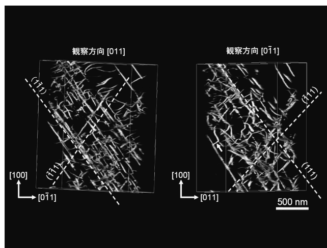
図6 直交する [011] および [0\bar{1}1] 方向から見た図5(c)の3次元再構成像。 \{111\} すべり面上の転位が直線状に観察されている。異なるすべり面間を移動する転位も見られる(矢印)。
