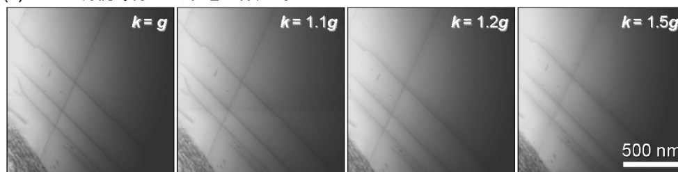
図3 TEM 明視野法(a)と STEM 明視野法(b)で撮影したフェライト( \alpha -Fe)中の転位像における回折条件依存性の比較。 g(hkl) = 310_{\alpha\text{-Fe}} の2波励起条件( k=g , k は散乱ベクトル)から励起誤差が正の方向に徐々に回折条件をずらしている。
