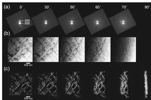
図5 オーステナイト系ステンレス鋼のSTEMトモグラフィ観察の例。(a) g(hkl)=200_{\gamma\text{-Fe}} の2波励起条件で撮影した連続傾斜電子回折図形の一部。図中の数値は試料傾斜角度。(b) (a)の各回折条件で撮影した転位の連続傾斜STEM明視野像の一部。(c) (b)の連続傾斜像から再構成した3次元転位像を、(a)や(b)と同様の方向から見たもの
