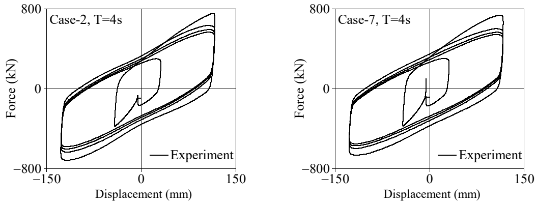
図 2.28 繰返し加力前後での基本特性試験の水平力-水平変位関係 (試験条件 2, 7)
