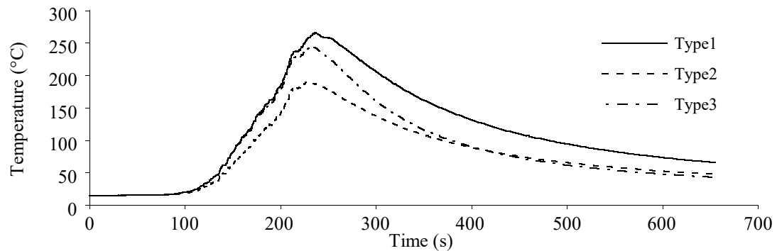
図 2.49 鉛プラグ中心温度の応答解析結果（長周期地震動(CH1)）
