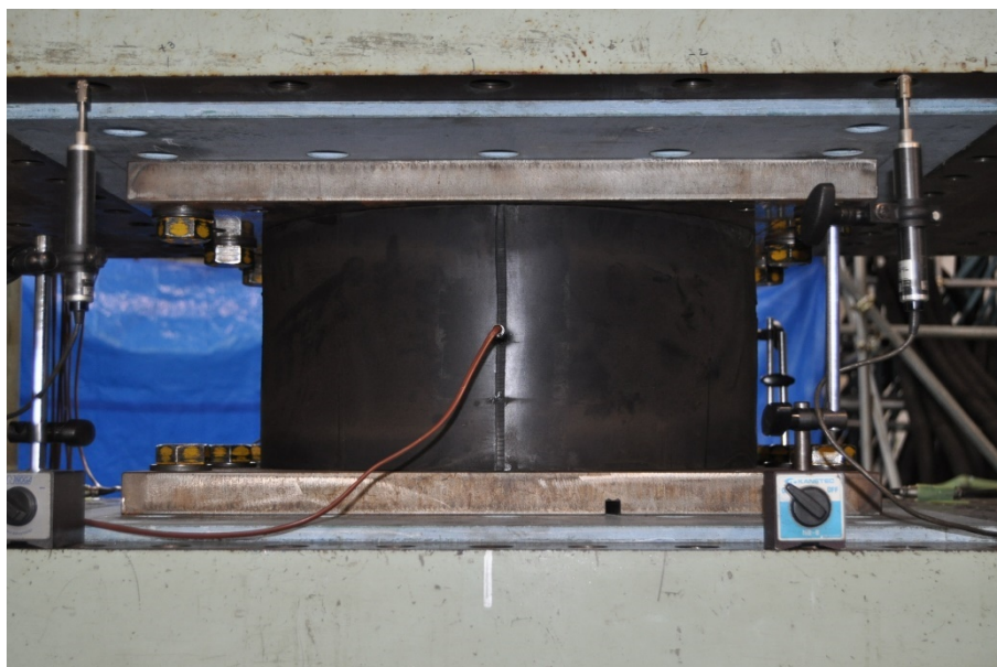
写真 3.1 LRB \phi 500 試験体
