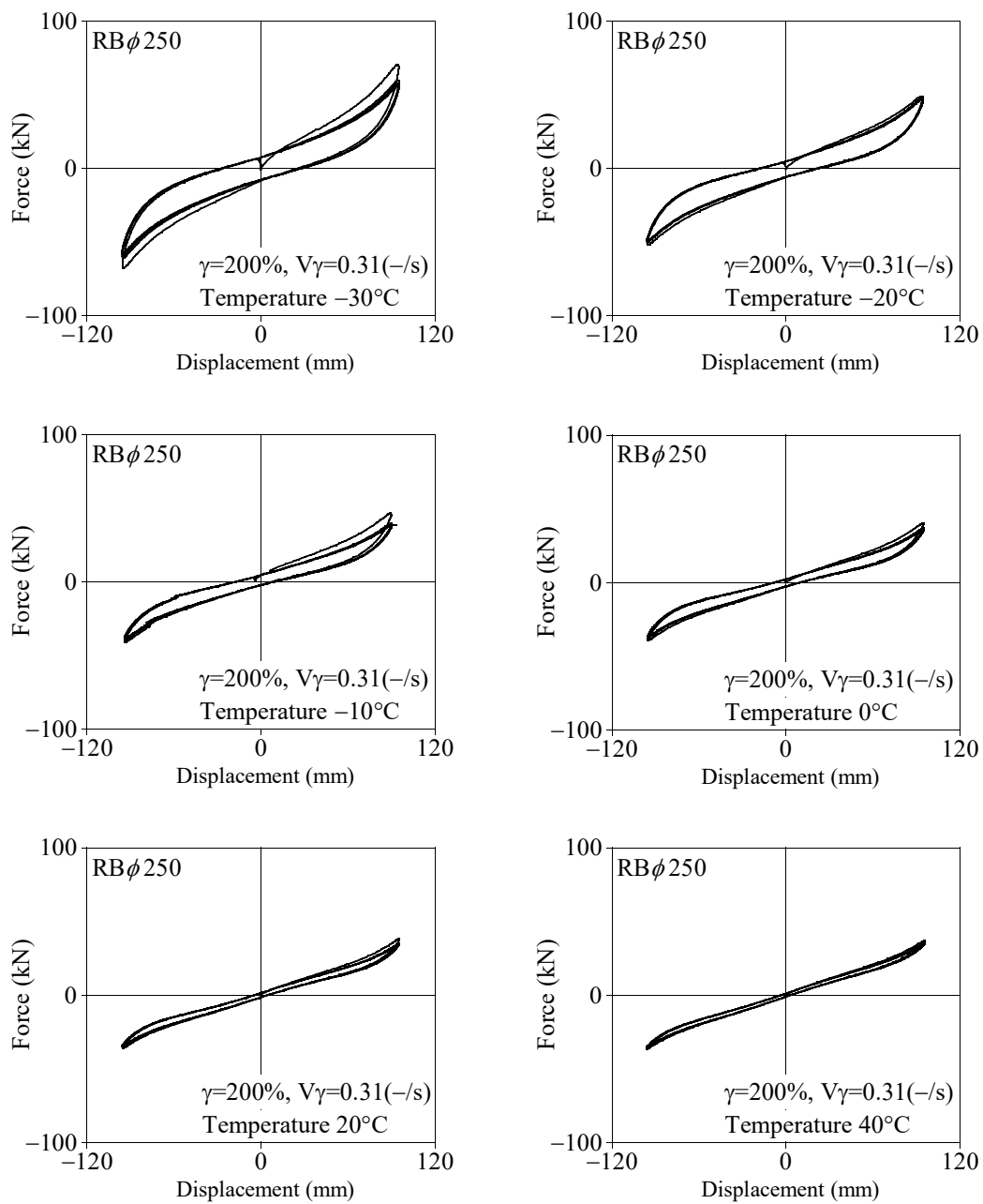
図 3.8 RB φ 250 試験体の水平力-水平変位関係 ( \gamma=200\% , V\gamma=0.31(-/s) ( T=40s ), Temp= -30, -20, -10, 0, 20, 40^{\circ}\text{C} )
