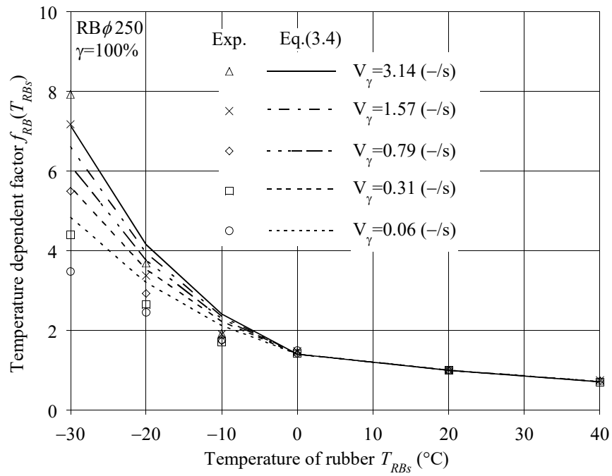
図 3.9 RB セン断応力度の温度依存性 ( \gamma=100\% )
