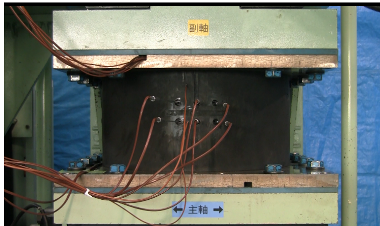
写真 2.1 Type-1 試験体
