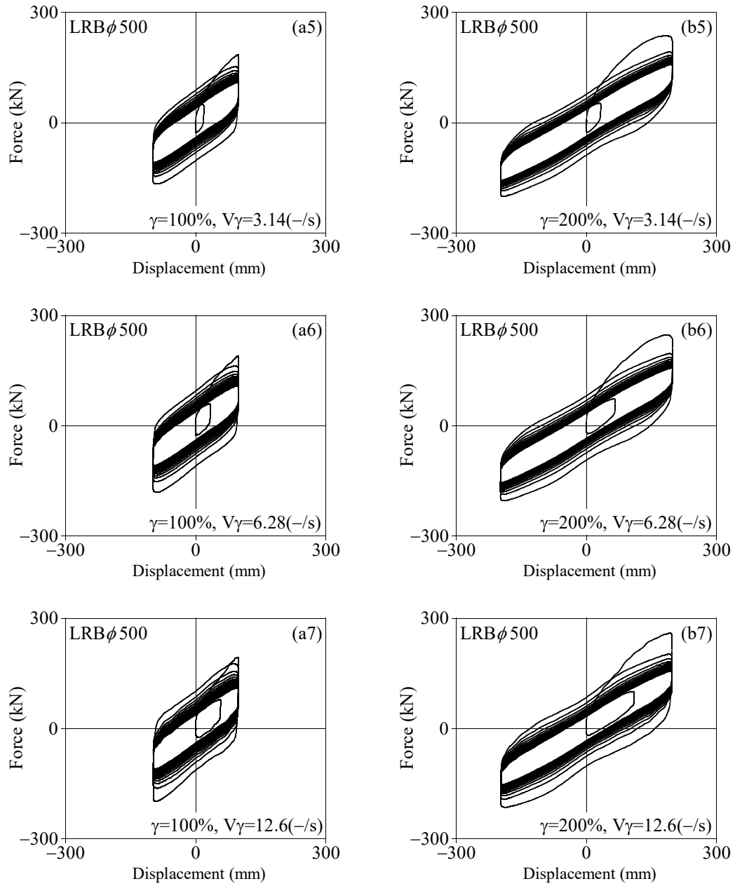
図 3.13 LRB \phi 500 速度依存性試験結果 (a) \gamma=100\% , (b) \gamma=200\%
