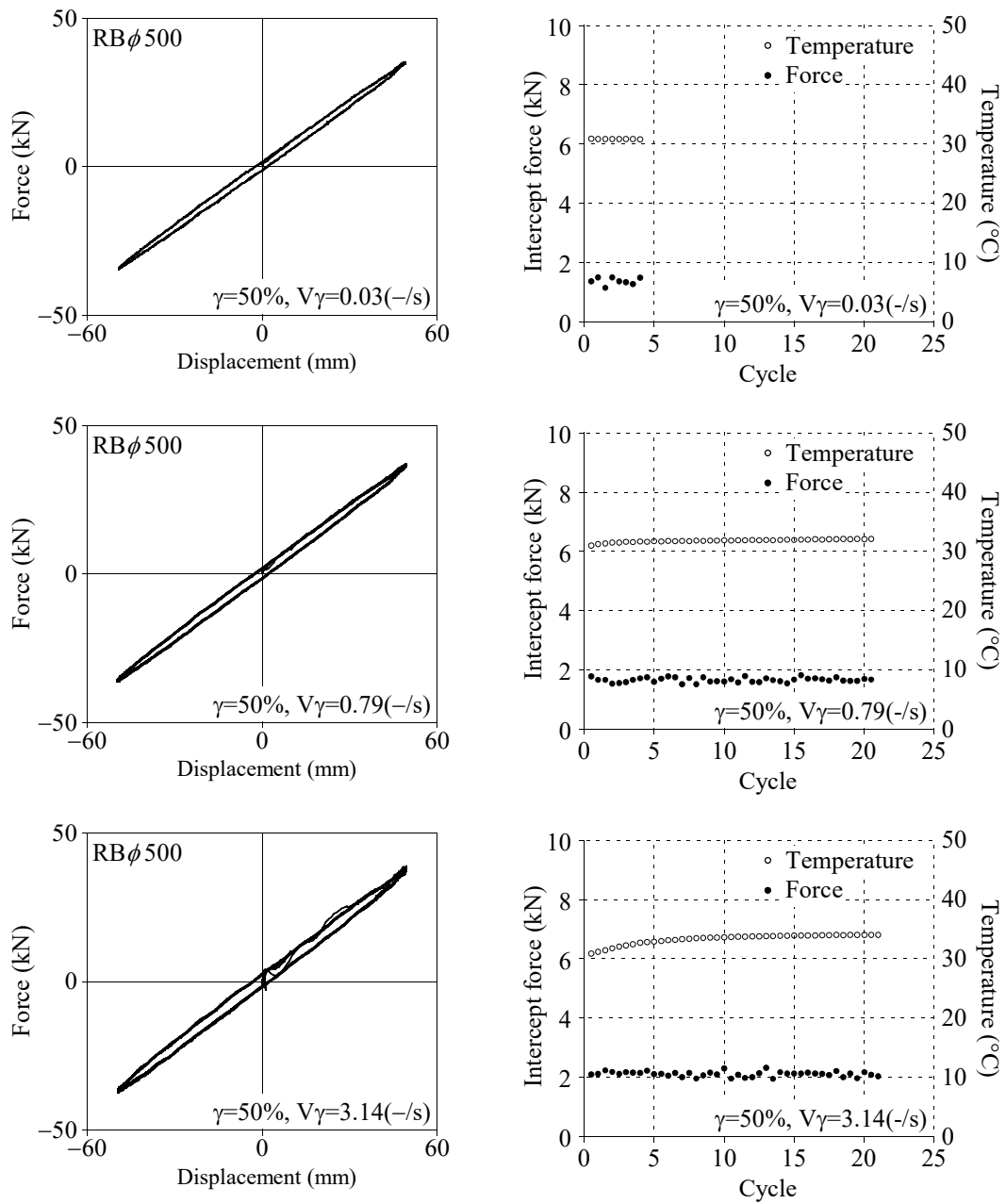
図 3.4 RB ϕ 500 試験体の水平力-水平変位関係と加力サイクルごとの RB 切片荷重と内部ゴム温度の関係 ( \gamma=50\% , V\gamma=0.03, 0.79, 3.14 (-/s))
