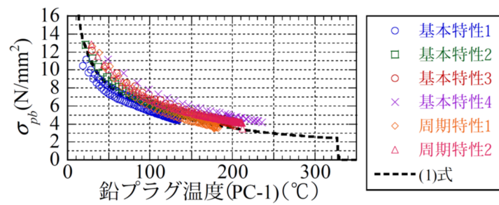
鉛プラグの温度と降伏せん断応力度の関係
