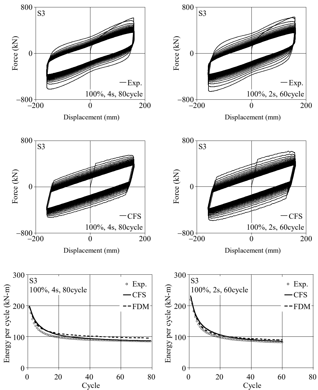
図 4.33 セン断ひずみ 100%, 加力周期 4s と 2s における 実験結果と CFS, FDM 解析結果
