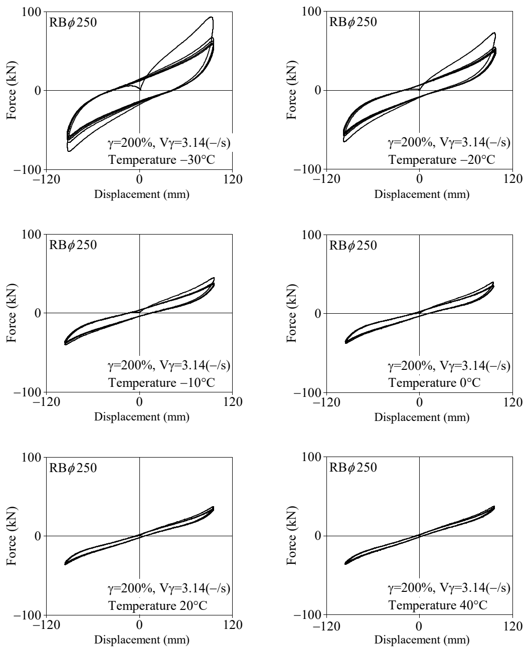
図 3.7 RB \phi 250 試験体の水平力-水平変位関係 (\gamma=200\%, V_{\gamma}=3.14 (-/s) \quad (T=4s), \text{Temp} = -30, -20, -10, 0, 20, 40^{\circ}\text{C})
