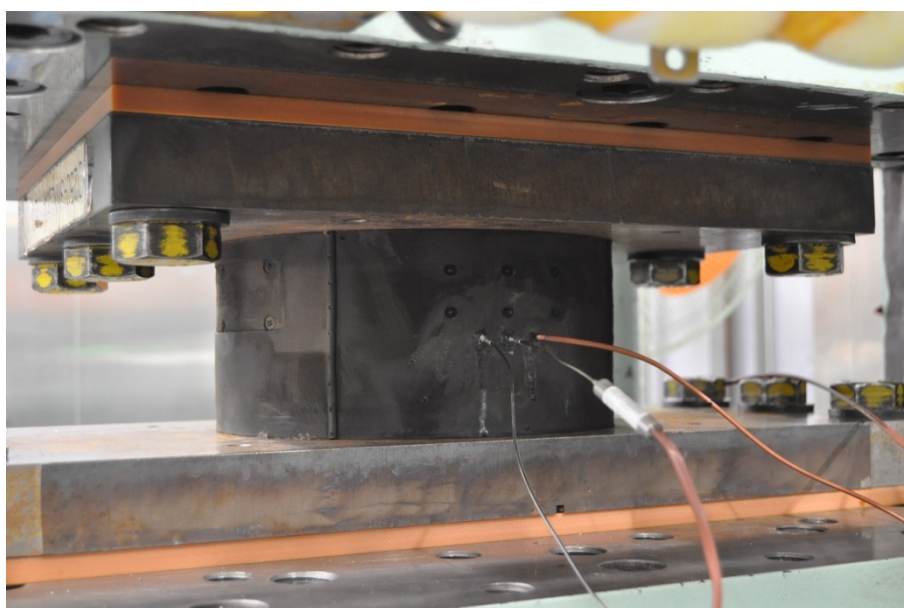
写真 3.2 LRB \phi 250 試験体
