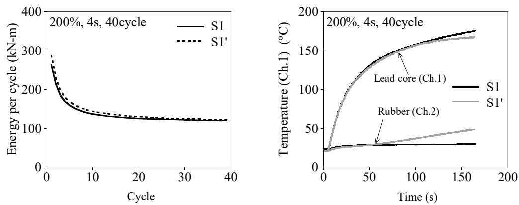
図 4.13 試験体 S1' と試験体 S1 の加力サイクル当たりのエネルギー吸収量と内部温度の変化
