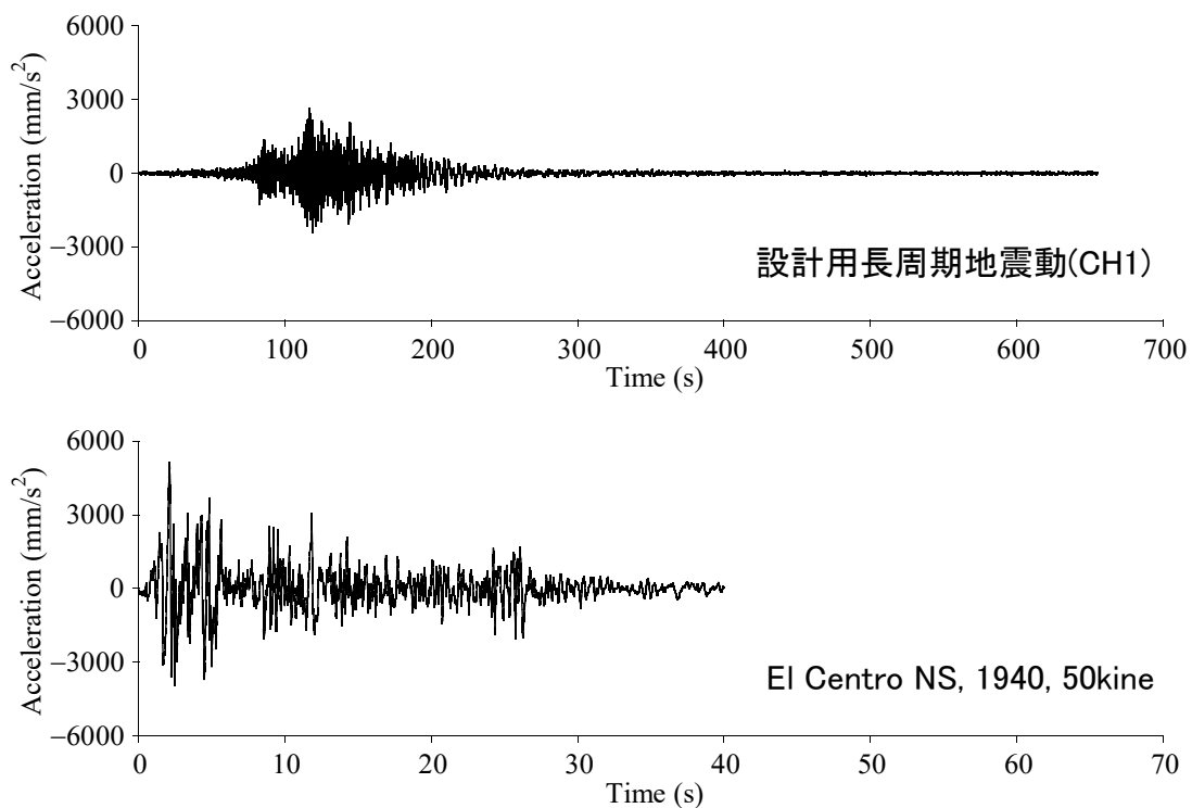
図 2.46 入力地震動
