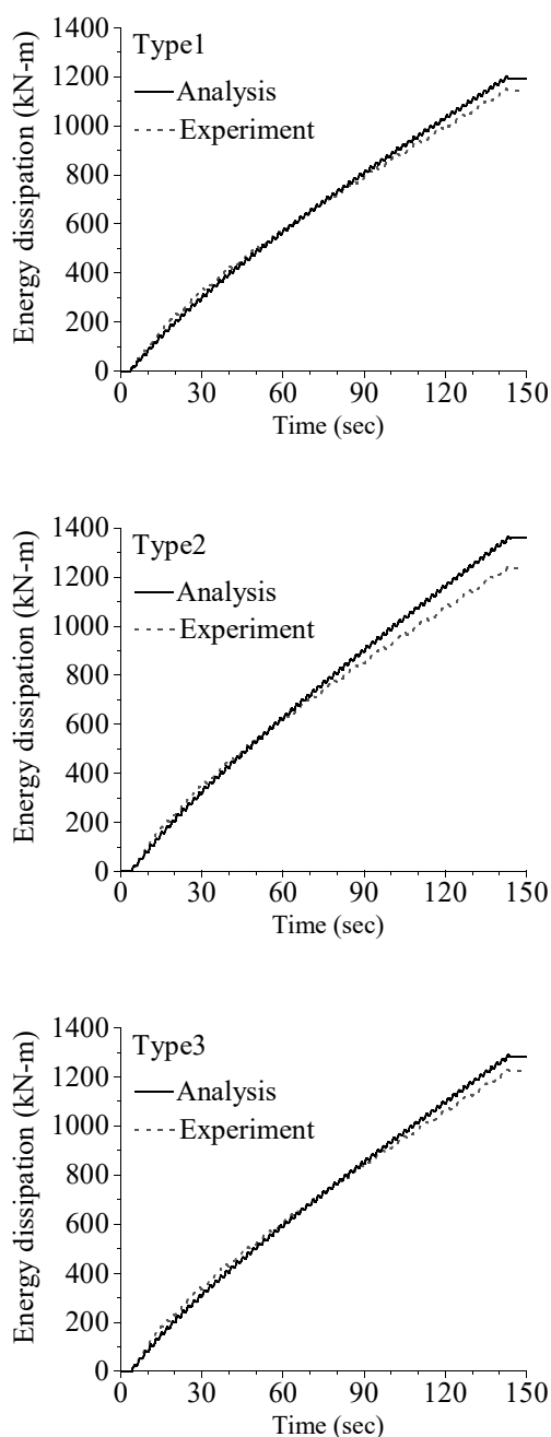
図 2.41 \gamma 200%試験における累積エネルギー吸収量と加力サイクルごとのエネルギー吸収量の実験結果と解析結果の比較（試験条件 2）
