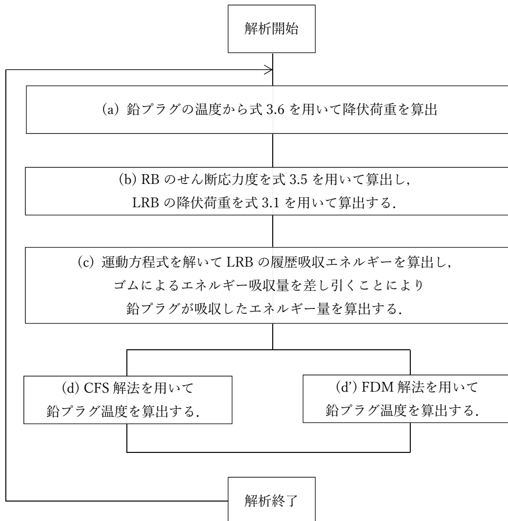
図 3.26 積層ゴムの非線形性を考慮した LRB の熱力学連成挙動解析の解析フロー
