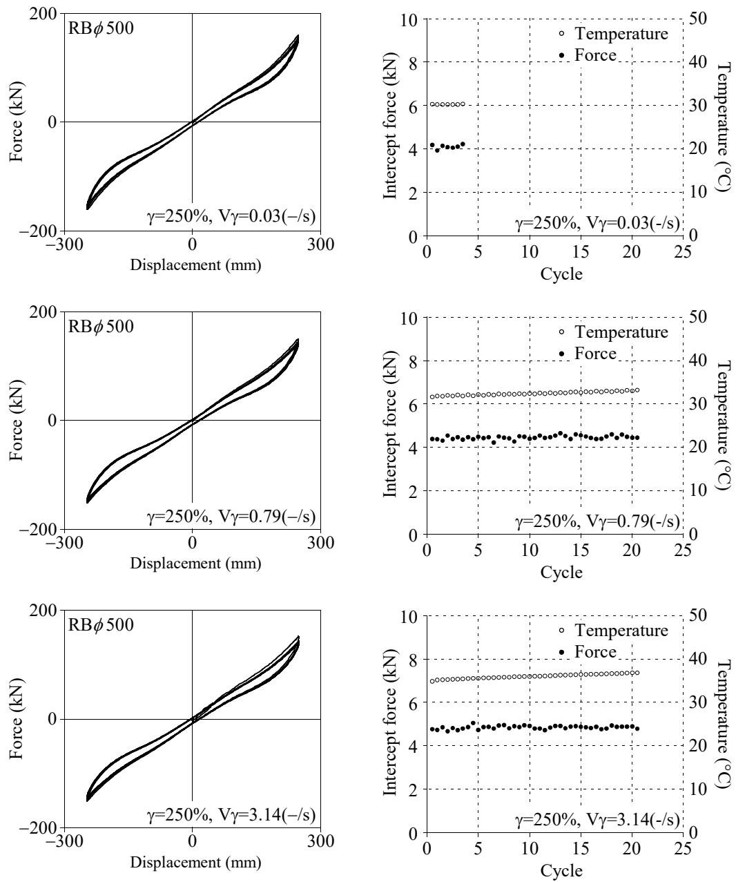
図 3.5 RB \phi 500 試験体の水平力-水平変位関係と加力サイクルごとの RB 切片荷重と内部ゴム温度の関係 ( \gamma=250\% , V\gamma=0.03, 0.79, 3.14 (-/s))
