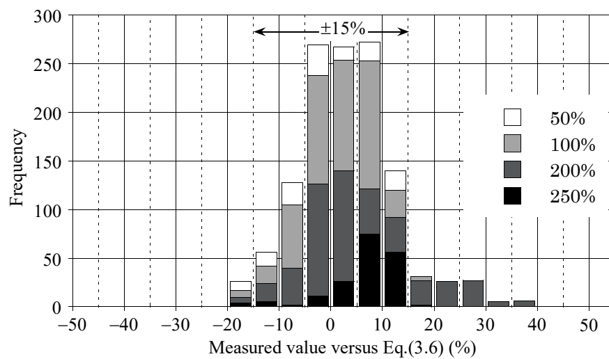
図 3.23 実験から得られた鉛プラグ降伏応力度の評価式 3.6 に対するばらつきのヒストグラム
