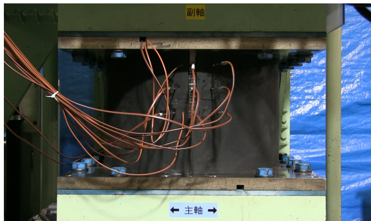
写真 2.2 Type-2 試験体
