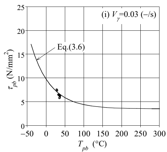
図 3.22 鉛プラグの降伏応力度と鉛プラグ中心温度の関係 ( V_\gamma=0.03 (-/s))
