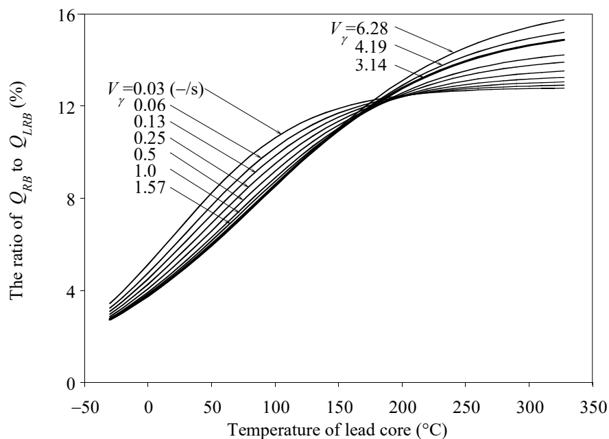
図 3.24 LRB 降伏荷重に与える RB セン断応力度の影響
