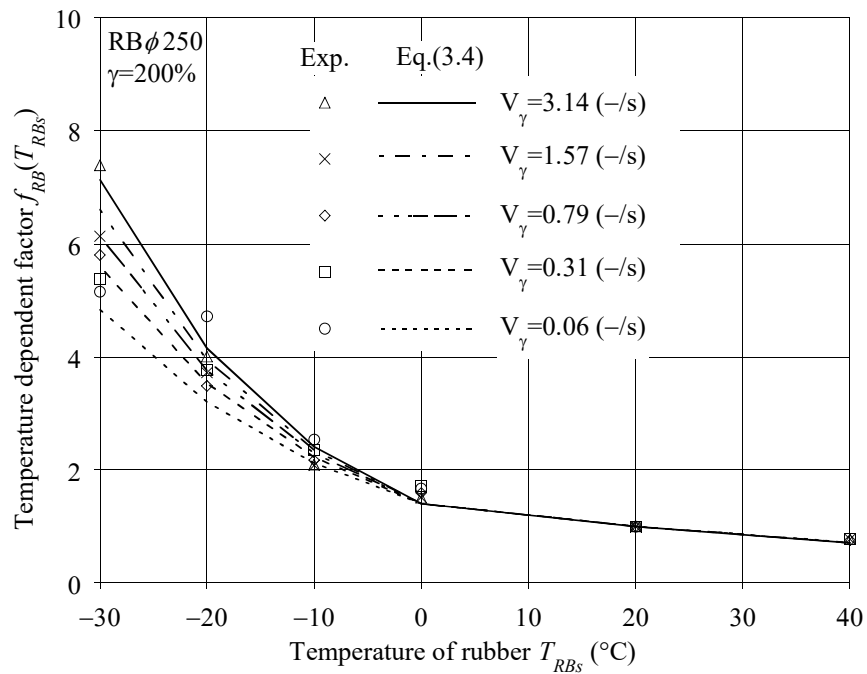
図 3.10 RB セン断応力度の温度依存性 ( \gamma=200\% )
