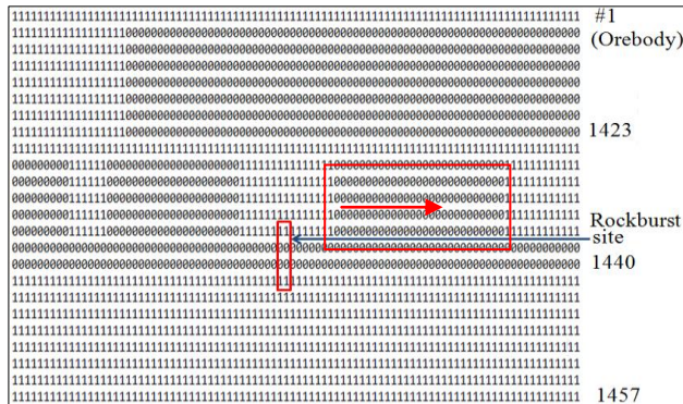
図3 坑道のレイアウト(0 既採鉱 1 未採鉱)
