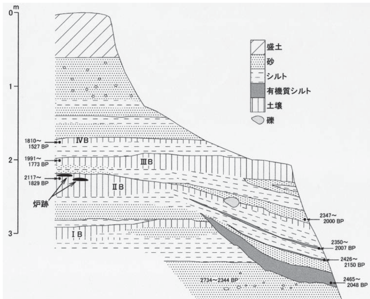
図3 文学部総合研究棟建設予定地土層断面
