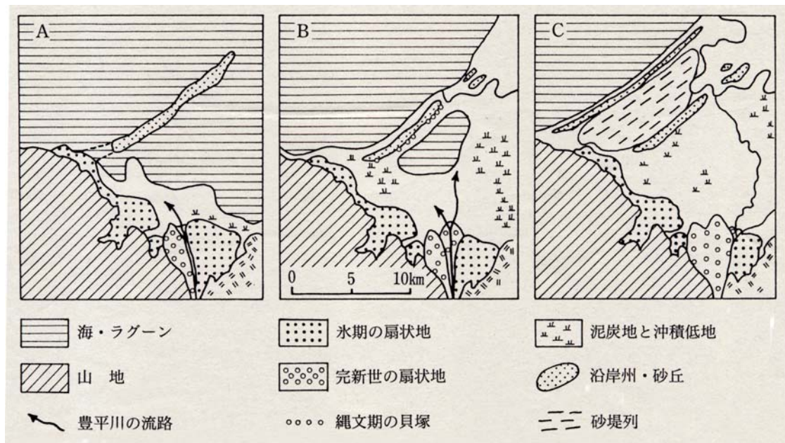
図4 縄文海進最盛期以降の札幌周辺の古地形の変遷
