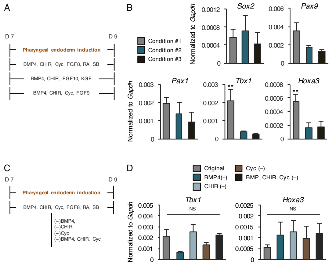
図7. AFE から PE の分化誘導と表現型解析
