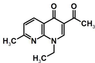
Nalidixic acid
