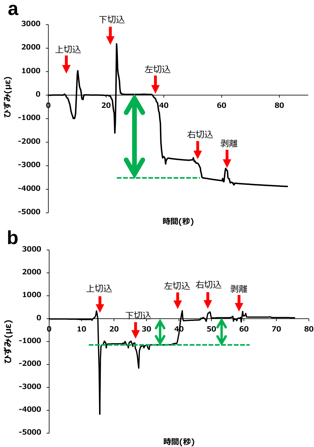
Fig. 4-17 ウダイカンバ(DBH=43 cm)外樹皮の解放ひずみ試験結果(a: 接線方向, b: 軸方向). 両矢印: Fig. 18, 19で示すひずみの量.
