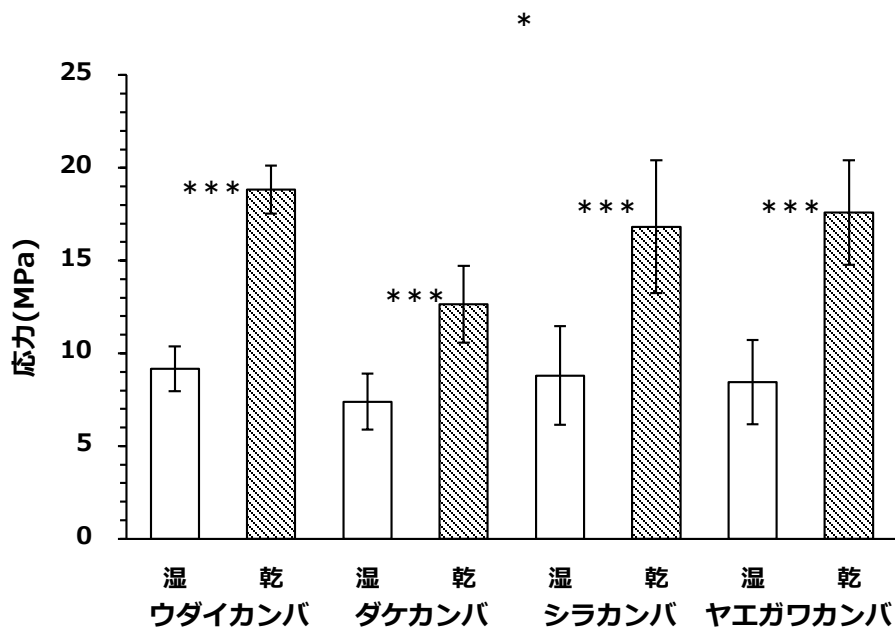
Fig. 4-6 湿潤試料と乾燥試料における引張最大応力(接線方向引張). エラーバーは標準偏差を示す. ***: p < 0.001 , t検定.
