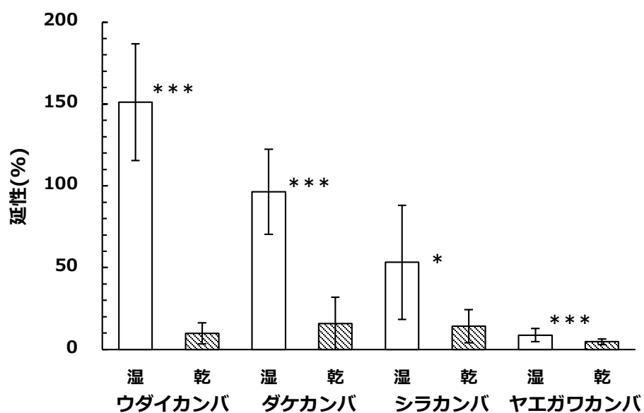
Fig. 4-3 外樹皮の湿潤試料と乾燥試料における延性(接線方向引張). エラーバーは標準偏差を示す. * : p < 0.05 , *** : p < 0.001 , t検定.
