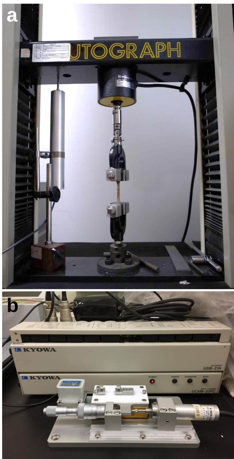
Photo 4-1 a: 縦引張試験機 AUTOGRAPH AGS-500D, b: 横引張試験機(手前)とデータロガー UCAM-20PC(奥).
