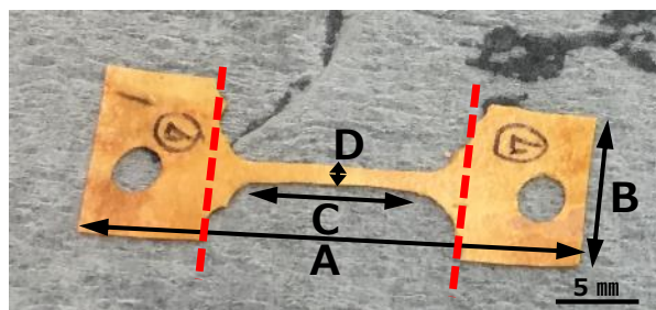
Fig. 4-2 試験体のサイズ：全長(A)：30 mm、両端の幅(B)：10 mm、平行部長さ(C)：10 mm、平行部幅(D)：1 mm。ヤエガワカンバの引張試験、ウダイカンバの応力緩和試験で使用。赤破線：つかみ部分。
