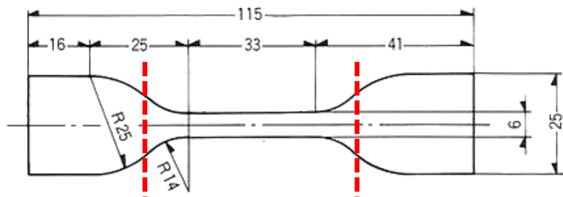
Fig. 4-1 試験体のサイズ：全長：115 mm、両端の幅：25 mm、平行部長さ：33 mm、平行部幅：6 mm。ウダイカンバ、ダケカンバ、シラカンバで使用。赤破線：つかみ部分。
