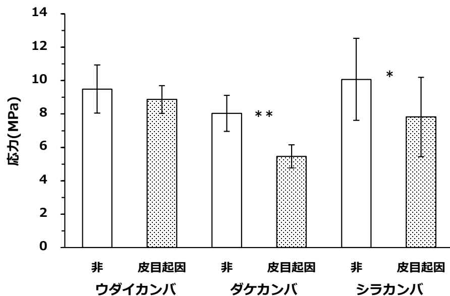
Fig. 4-9 皮目のない部位で破断した試料(非)と皮目から破断した試料(皮目起因)における引張最大応力(接線方向引張). エラーバーは標準偏差を示す. *: p < 0.05 , **: p < 0.01 , t検定.
