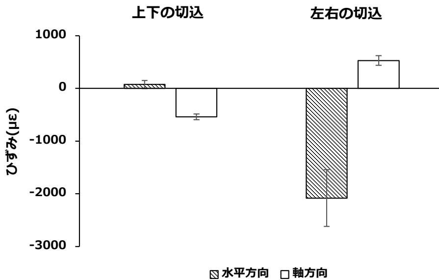
Fig. 4-19 シラカンバ幹 (DBH=18.5 cm) 外樹皮の解放ひずみ試験結果. n=6(水平方向)、n=3(軸方向). エラーバーは標準偏差を示す.
