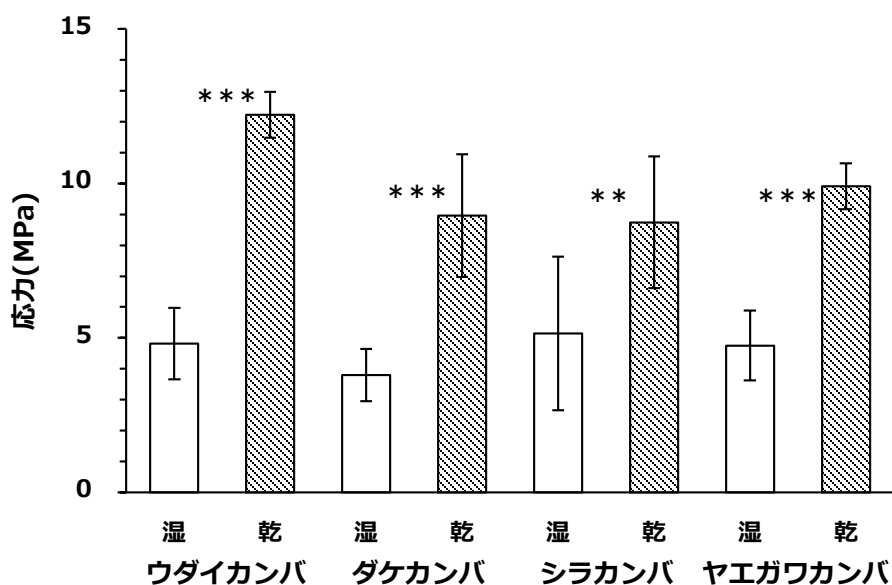
Fig. 4-5 湿潤試料と乾燥試料における引張比例限度応力(接線方向引張). エラーバーは標準偏差を示す. **: p < 0.01 , ***: p < 0.001 , t検定.
