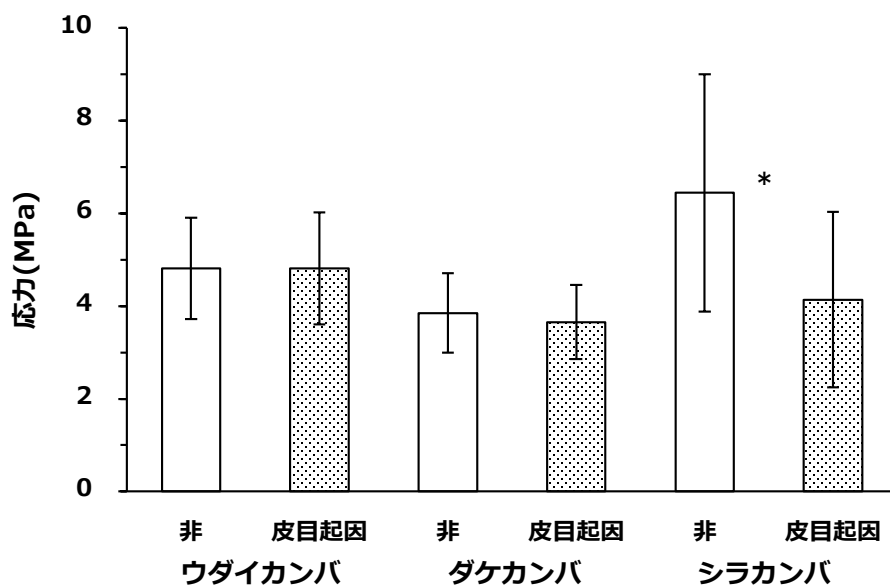
Fig. 4-8 皮目のない部位で破断した試料(非)と皮目から先行破断した試料(皮目起因)における引張比例限度応力(接線方向引張). エラーバーは標準偏差を示す. *: p < 0.05 , t検定.
