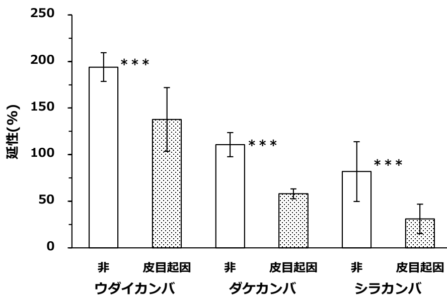
Fig. 4-7 皮目のない部位で破断した試料(非)と皮目から先行破断した試料(皮目起因)における延性(接線方向引張). エラーバーは標準偏差を示す. *** : p < 0.001 , t検定.
