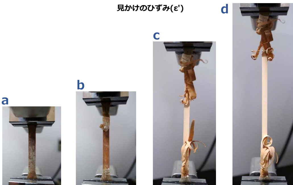
Fig. 4-4 ウダイカンバ外樹皮の湿潤試料と乾燥試料の応力-ひずみ曲線(接線方向引張)と湿潤試験体の各引張過程の様子. a: 弾性域でまだ変形していない様子. b: 最外層が破断した様子. c: 内層部分がよく伸びる様子. d: 内層が破断する直前の様子.
