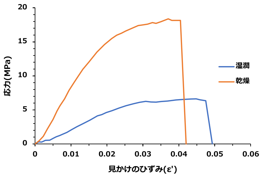
Fig. 4-11 ヤエガワカンバ外樹皮の湿潤試料と乾燥試料の応力-ひずみ曲線(接線方向引張).
