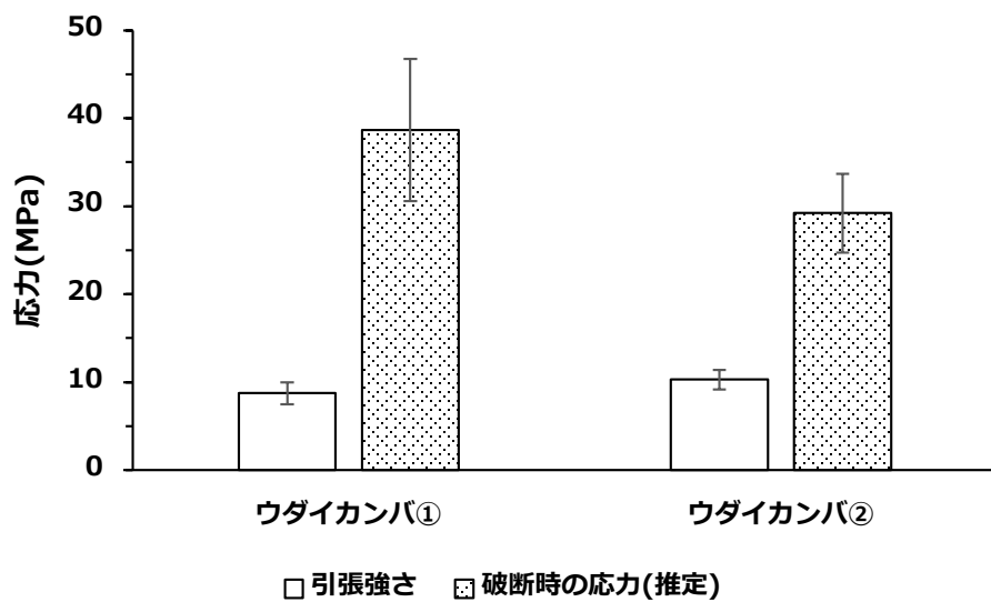
Fig. 4-16 ウダイカンバ外樹皮の見かけの断面積から計算した場合の最大応力(引張強さ)と破断時の断面積から推定した破断時の応力(接線方向引張). エラーバーは標準偏差を示す.
