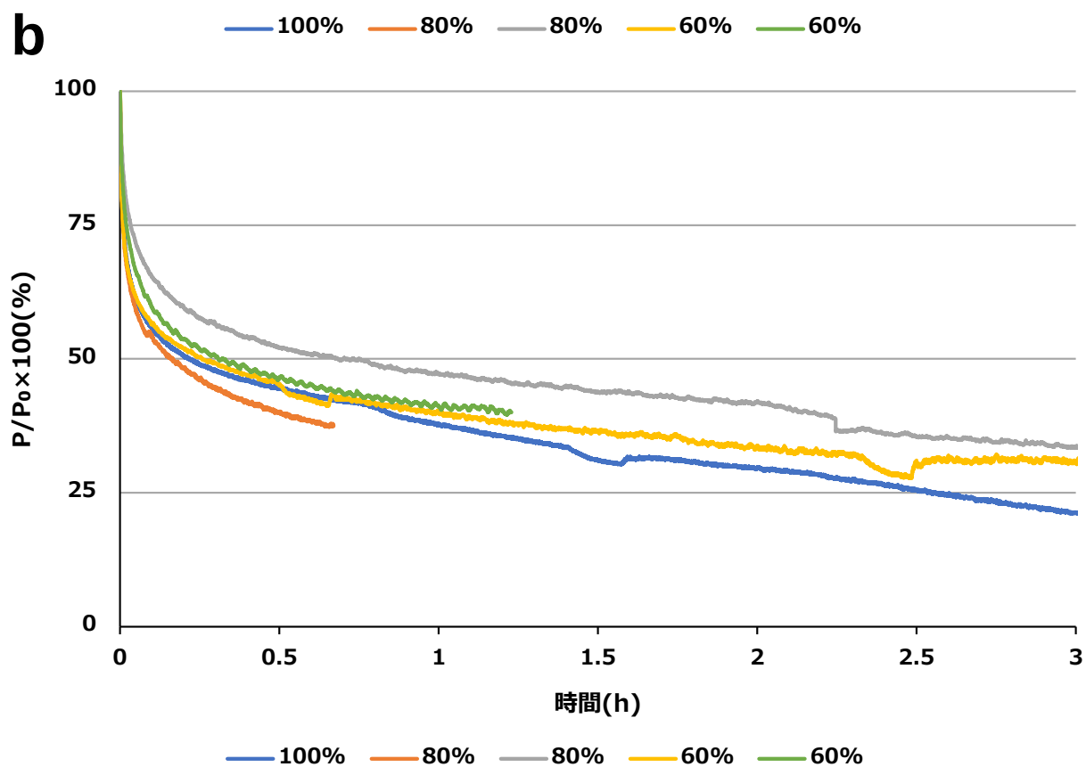
Fig. 4-20 ウダイカンバ(DBH=42 cm)外樹皮の応力緩和試験結果. 各数値(%)は比例限度におけるひずみに対する初期ひずみの割合を示す. a: 時間(h)の最大値は17時間. b: aの一部(赤点線囲い)の拡大で、時間(h)の最大値は3時間.
