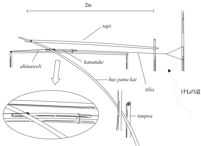
図3 イノシシ、シカを捕獲するための槍罠 (hus pana)
