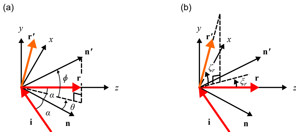
図 C.1 2 軸可動鏡での入射・反射における各ベクトル・角度の定義。(a) 2 軸可動鏡の法線ベクトルの回転。(b) 反射光線ベクトルの回転。 z 軸は 2 軸可動鏡とその下流のレンズペアそれぞれの中心を通る。2 軸可動鏡の法線ベクトルを方位角方向、仰角方向にそれぞれ \theta, \phi 回転させると反射光線ベクトルは元の状態（図中赤色のベクトル \mathbf{r} ）から方位角方向、仰角方向にそれぞれ \zeta_r, \zeta_r 回転する（図中橙色のベクトル \mathbf{r}' ）。
