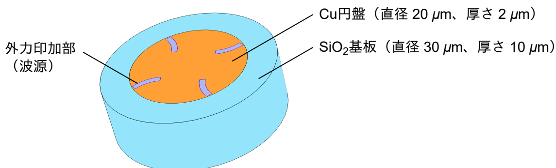
図 2.19 WGM シミュレーションの系。橙色の領域が銅製円盤、水色の領域が円柱状の SiO 2 基板である。Cu 円盤の直径と厚さはそれぞれ 20 \mu\text{m} 、 2 \mu\text{m} であり、SiO 2 基板の直径と厚さはそれぞれ 30 \mu\text{m} 、 10 \mu\text{m} である。円盤表面の紫色の円弧型の 4 個の部分で波源となる。この部分に対し、媒質表面に垂直に外力を印加する。
