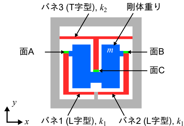
図 3.23 単位構造の面外曲げ共振モードの準解析モデル。青色と赤色の領域それぞれが構造内部の剛体重り、捻りバネとなる。バネ 1, 2 は L 字型、バネ 3 は T 字型をしている。重りは紙面の面外方向に振動する。緑色の部分は各バネの先端の面を示す。灰色の外枠部分は変位しない剛体である。
