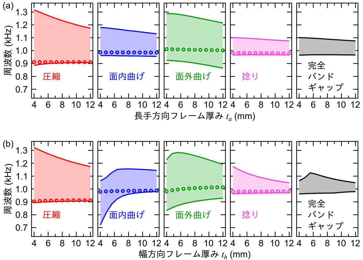
図 3.8 局所共振モードの周波数とバンドギャップの t_a, t_h 依存性。(a) t_a 依存性。(b) t_h 依存性。 t_a, t_h とともに初期値（前述の各シミュレーションで使用した値）は 8.0 mm である。実線が各バンドギャップのギャップ端、網掛け部分がバンドギャップの帯域、丸印が対応する局所共振モードの周波数を示す。
