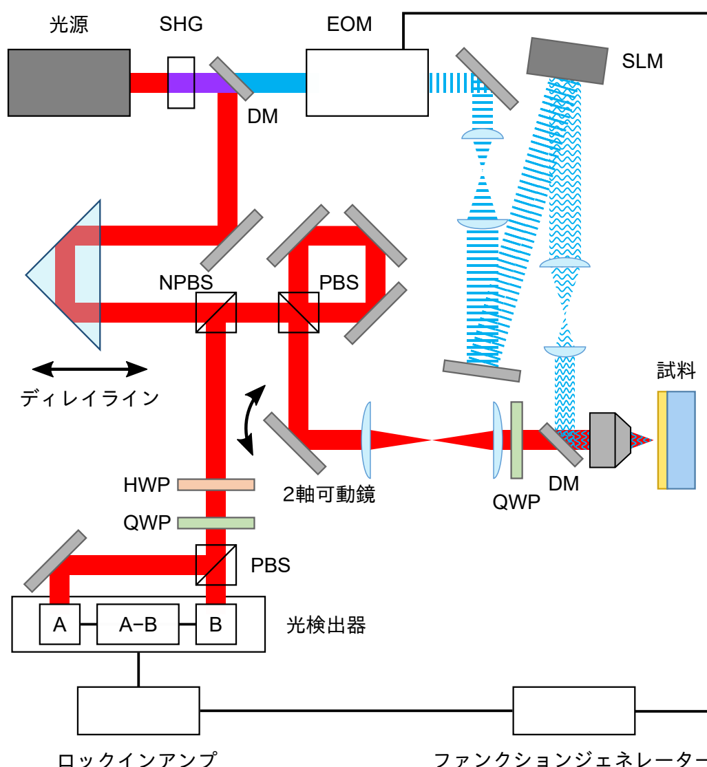
図 2.10 実験に用いた光学系の概略図。主な点は図 2.1 と同様である。ポンプ光は EOM で時間的な強度変調を、SLM で空間的な位相変調を受けてから試料に入射する。プローブ光はディレイライン、干渉計、2 次元走査系を経て試料に入射し、試料で反射された後に光検出器へ向かう。
