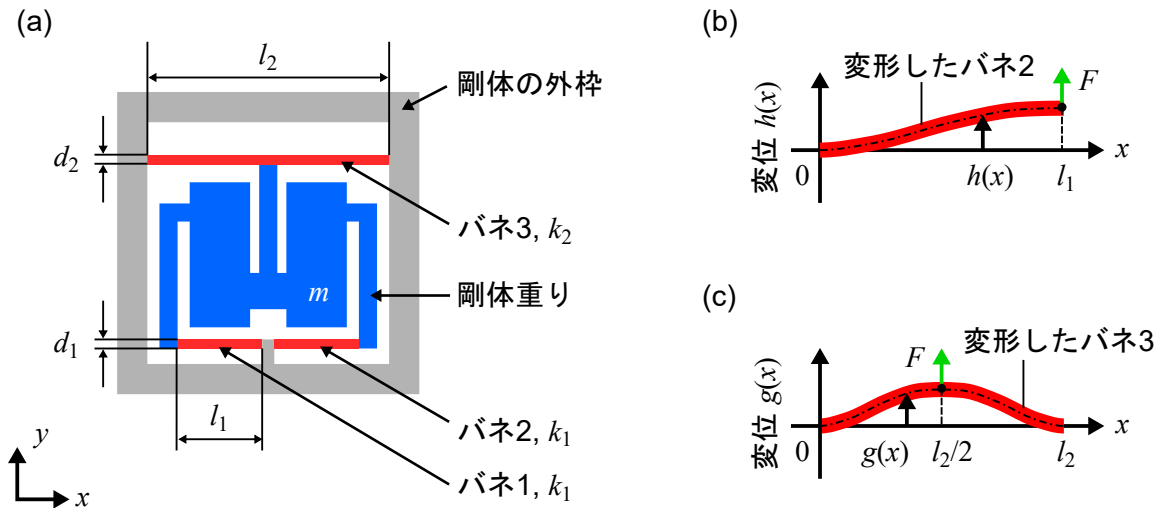
図 3.20 単位構造の圧縮共振モードの近似的解析モデル。(a) モデル化した単位構造。青色と赤色の領域それぞれが構造内部の剛体重り、曲げバネ（板バネ）となる。重りは梁の長手方向に振動する。灰色の外枠部分は変位しない剛体である。(b) バネ 2 に外力 F を働かせたときのバネの変形の様子。赤色の曲線が変形したバネを示す。黒色の一点鎖線がバネの中立面を示す。(c) バネ 3 についての同様の図。
