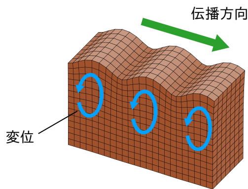
図 1.1 Rayleigh 波の模式図。青色、緑色の矢印はそれぞれ各点の変位方向、波の伝播方向を示す。表面近傍の各点が楕円を描くように振動しながら波が伝わる。
