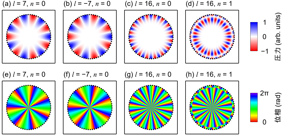
図 1.2 2次元系において円形の剛体の壁に囲まれた空気中を伝わる音響ウィスパーリングギャラリーモードの例。(a)-(d) それぞれ (l, n) = (7, 0), (-7, 0), (16, 0), (16, 1) の場合の音圧分布。(e)-(h) それぞれ (a)-(d) 同様のモードの位相分布。各図の黒い点線は空気と壁との境界を示す。壁の外側に音響場は漏れ出さないため、壁内部の空気中でのみ音圧と位相が定まる。(a) と (b) のように次数 l の絶対値が同じモードのある瞬間の音圧分布に差はなく、(e) と (f) のように位相の進む向きのみが異なる。
