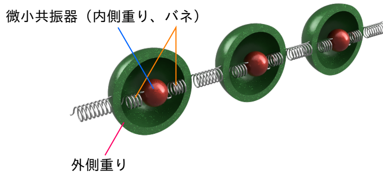
図 1.6 音響メタマテリアルの 1 次元重りバネモデルの模式図。系は周期的な重りとバネの組により構成される。単位構造は外側（緑色）の重り、内側（赤色）の重り、それぞれの重り同士をつなぐバネからなる。それぞれの重りは球形であるが、単位構造の内部を見やすいように外側重りは半分には切っている。
