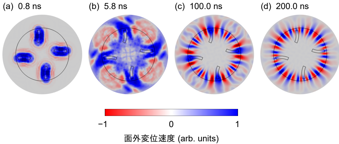
図 2.21 d = 1.0\ \mu\text{m} , \theta = 50^\circ の場合の媒質表面の面外変位速度の分布。(a)-(d) それぞれ 0.8 ns, 5.8 ns, 100.0 ns, 200.0 ns である。カラスケールは各時刻で適宜変更している。
