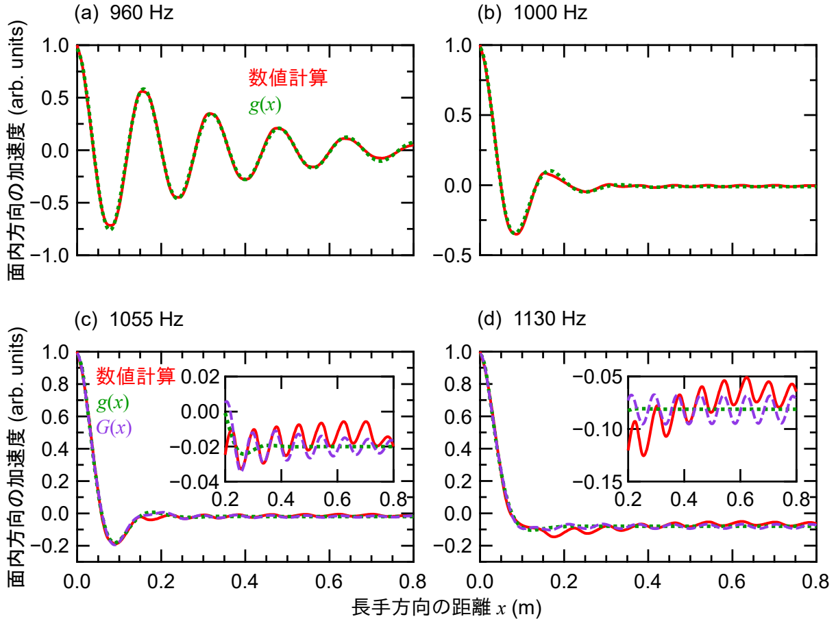
図 3.15 面内曲げモードにおける 10 ユニットのメタマテリアル梁の辺上での幅方向の加速度分布。(a)-(d) それぞれ 960 Hz, 1000 Hz, 1055 Hz, 1130 Hz の結果。(a)-(d) の赤色の実線と緑色の点線はそれぞれシミュレーション結果と関数 g(x) のフィッティング曲線を示す。(c) と (d) の紫色の破線は関数 G(x) でのフィッティング曲線を示す。(c) と (d) の内挿図はそれぞれのグラフの x = 0.2 m から x = 0.8 m までの範囲の拡大図である。
