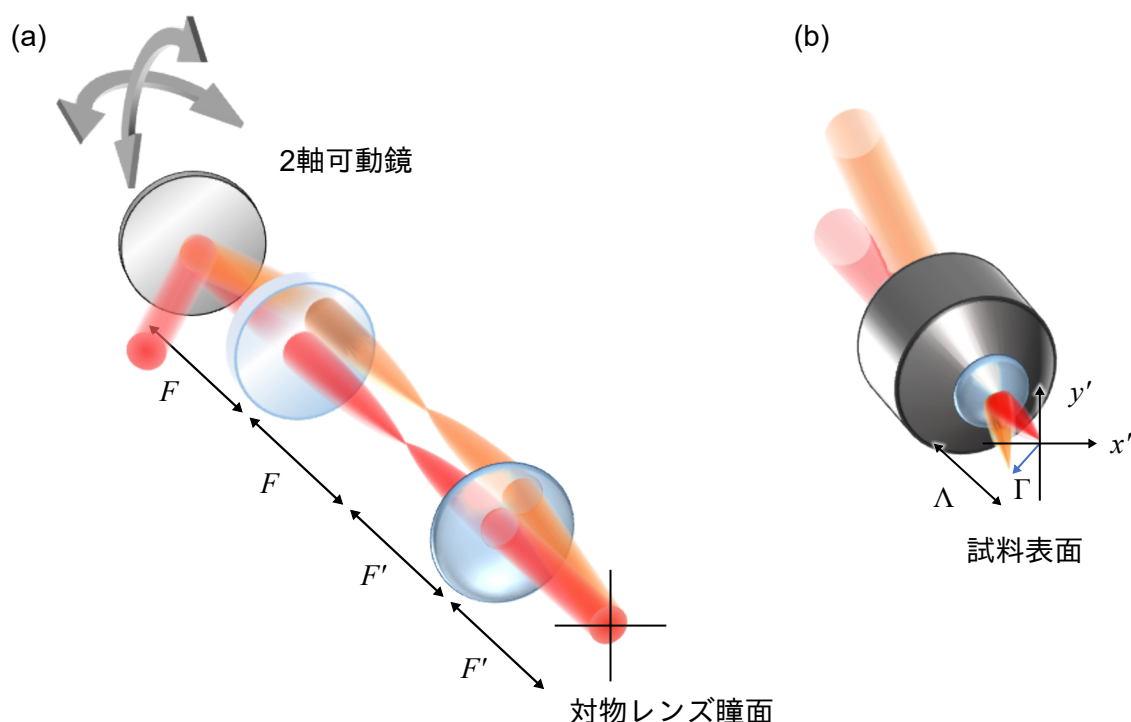
図 2.4 2次元走査を行う光学系の模式図。(a) 2軸可動鏡から対物レンズまで。(b) 対物レンズから試料まで。 F, F', \Lambda はそれぞれのレンズの焦点距離である。赤色と橙色はともにプローブ光を表し、それぞれ、2軸可動鏡の角度に応じた別々の経路を通る場合を示す。プローブ光の波長は実際には一定だが、ここでは便宜的にそれぞれの経路でプローブ光の色を変えている。(a) における灰色の矢印は2軸可動鏡の回転方向を示す。2軸可動鏡の角度を変えることで試料表面、すなわち、 x'y' 面におけるプローブ光の集光位置が \Gamma 動くため試料の2次元走査が可能となる。
