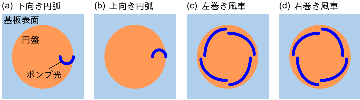
図 2.6 円弧型・風車型に集光したポンプ光の模式図。(a), (b) それぞれ互いに向きが反転している下向き円弧型・上向き円弧型ポンプ光。(c), (d) それぞれ互いに向きが反転している左巻き風車型・右巻き風車型ポンプ光。媒質は基板（水色）の上部に円盤（茶色）を埋め込んだ構造である。(a)-(d) それぞれのように円盤内でカイラルな強度分布となるようにポンプ光（濃い青色）を集光する。これによりポンプ光の集光形状と同様の形の波源を形成する。どの波源も円盤内での位置や形状の対称性が低くカイラルなため、縮退する WGM の内、一方が他方よりも強く励起される。また、(a), (b) の円弧型波源同士、(c), (d) の風車型波源同士で互いにカイラリティの向きが逆なため、それぞれの波源で強く生じる WGM も反対となる。
