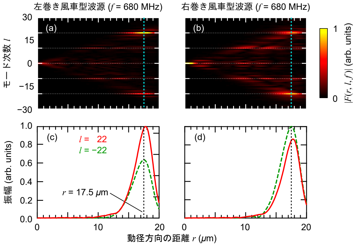
図 2.18 風車型波源を形成した場合の f = 680 \text{ MHz} における振幅絶対値 |F(r, l, f)| の分布。(a), (b) それぞれ左巻き風車型波源、右巻き風車型波源を形成した場合の rl 平面での振幅分布である。(c), (d) それぞれ (a), (b) の結果から l = \pm 22 のみを抜き出したグラフである。ただし、強く生じた方のモードの振幅最大値が 1 になるように双方の結果をスケールリングしている。赤色の実線と緑色の破線はそれぞれ l = 22, -22 の成分を示す。(a), (b) の青色の点線と (c), (d) の黒色の点線は r = 17.5 \mu\text{m} を示す。
