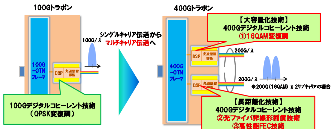
図 2.7: 400Gbps トランスポンダ(送信部)の構成
