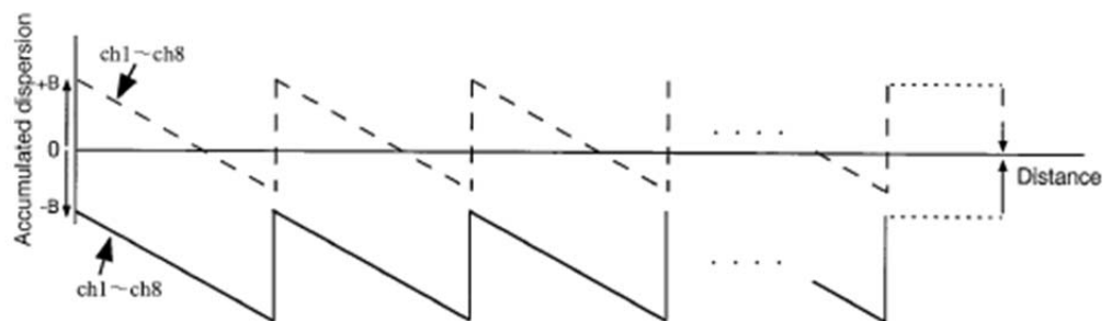
(d) Dispersion map in model 2
