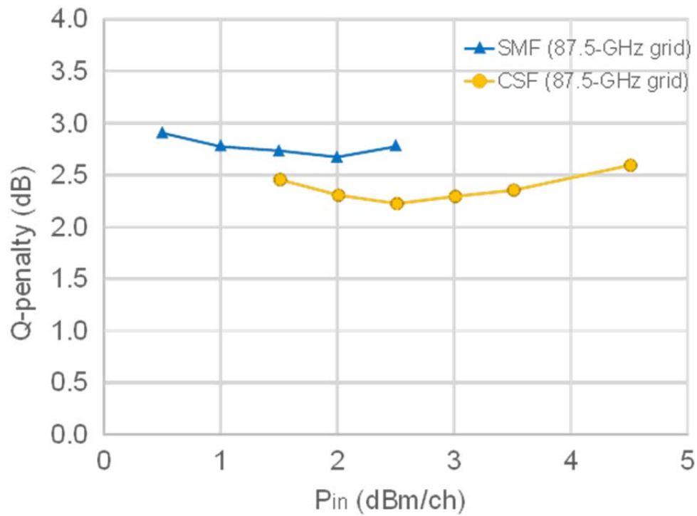
図 3.6 ファイバ入力パワーと Q ペナルティの関係
