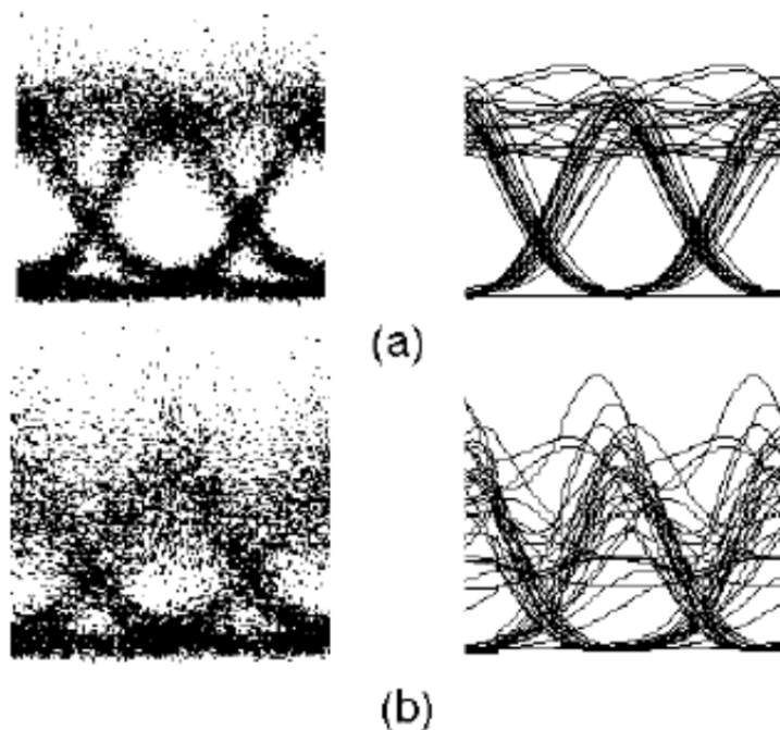
図 4.17: 受信波形
