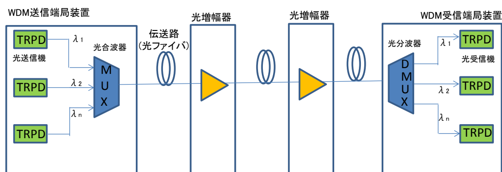
図 1.3: 波長多重光伝送システム
