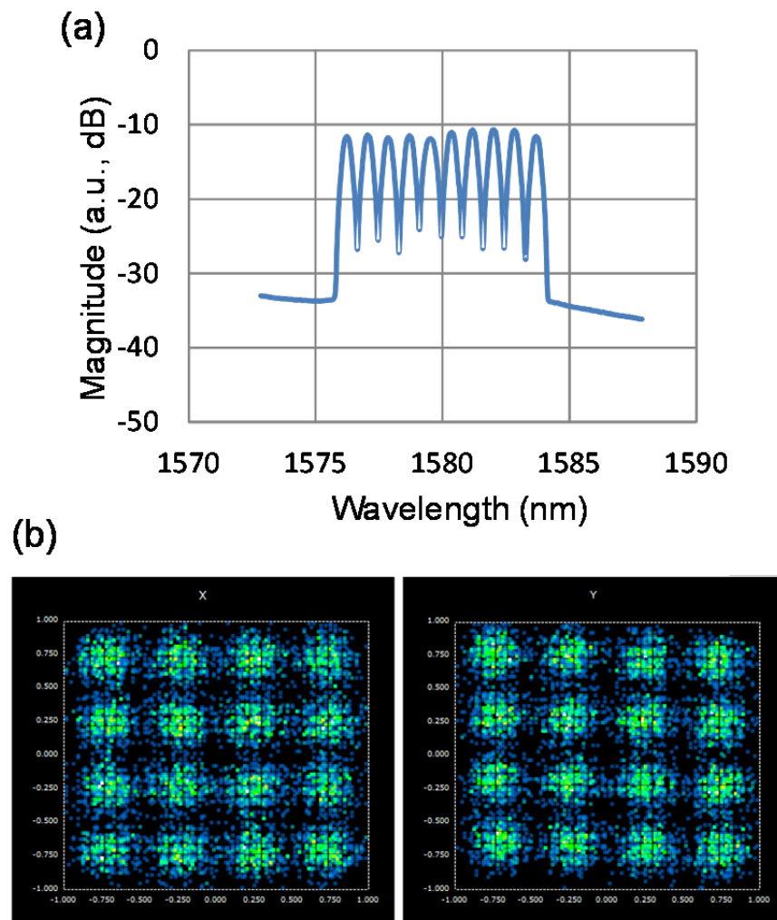
図 3.8 2,000km 伝送後のスペクトルとコンスタレーション
