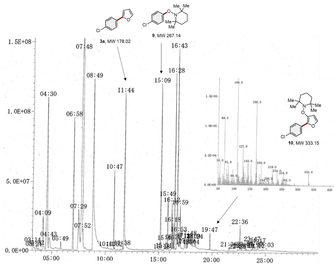
Fig. S4. The GC-MS chart.
