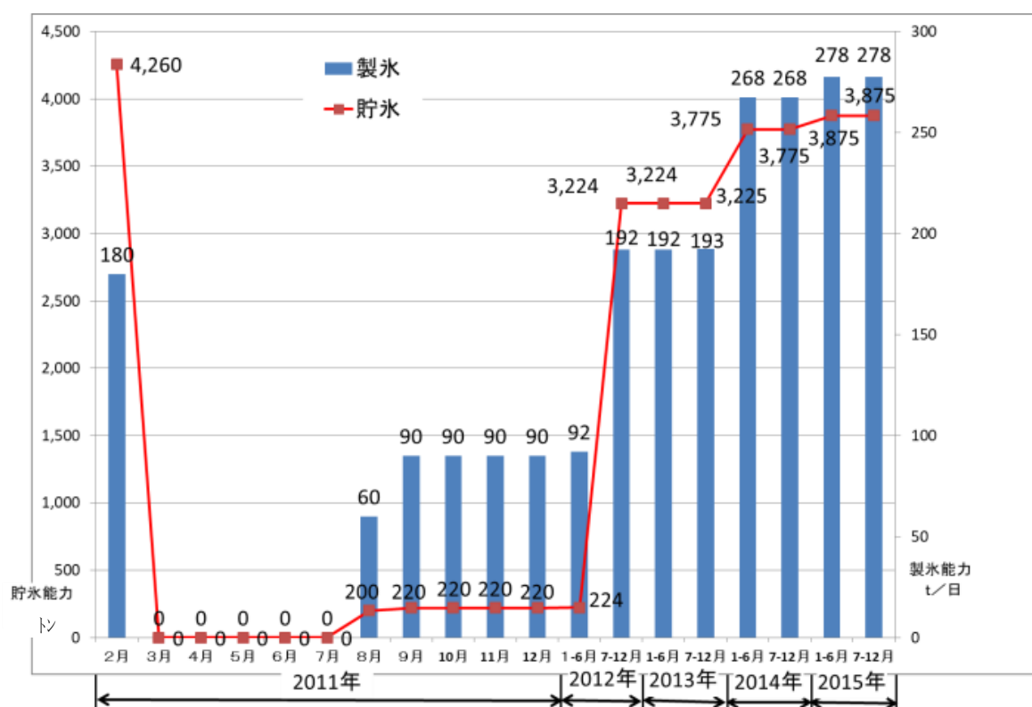
図4-8 製氷・貯氷機能の復旧過程 4)
