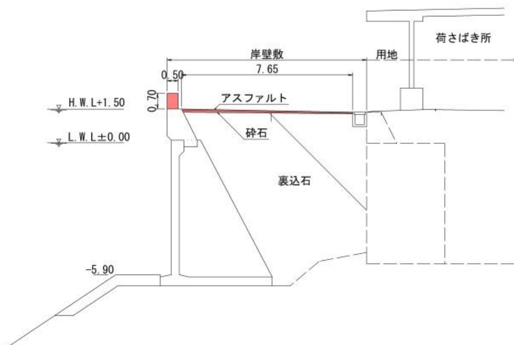
図 4-11 魚市場前岸壁の仮復旧工事標準断面図
