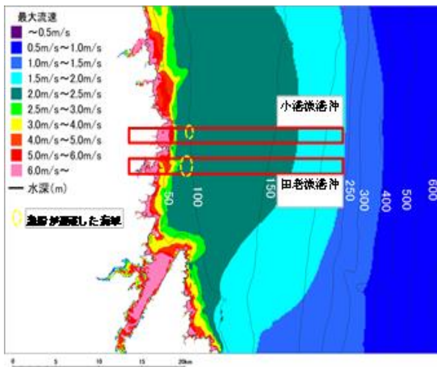
図 3-2-12 津波シミュレーションによる田老漁港周辺の最大津波流速分布
