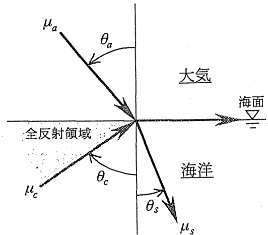
図2 入射放射の海面における屈折
