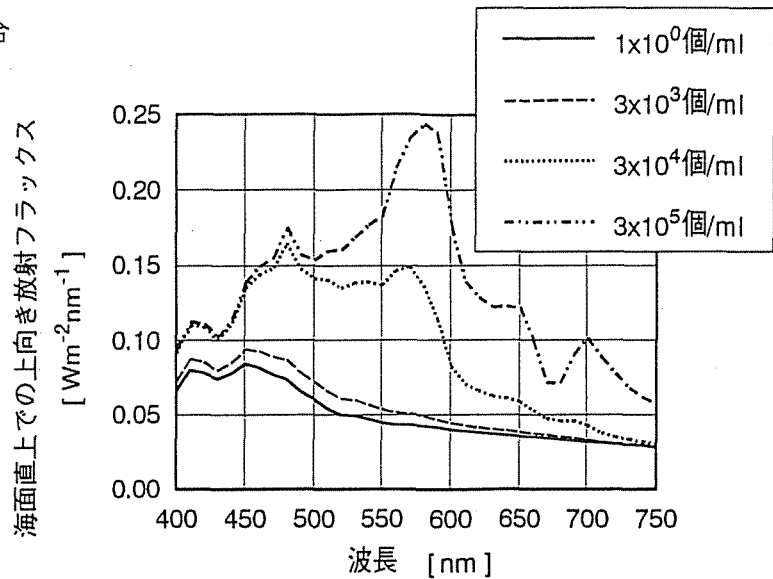
図8 デトリタスを伴う赤潮発生海域における海面直上での上向き放射フラックス
