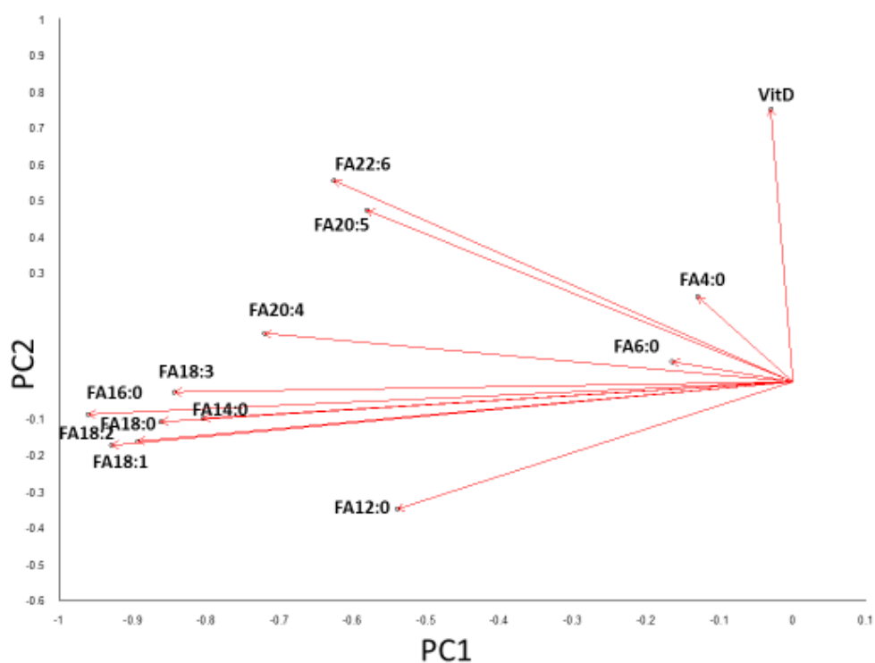
Fig.4.9 Result of free fatty acid dataset (PCA)
