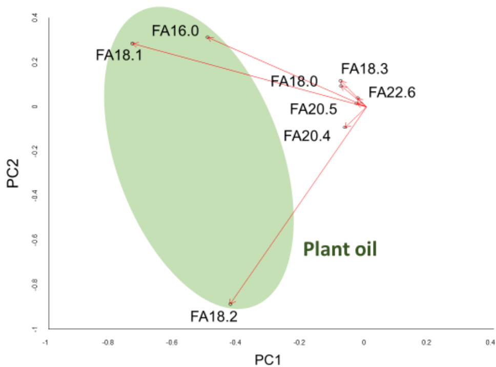
Fig.4.17 Result of fatty acid dataset (CPCA)
