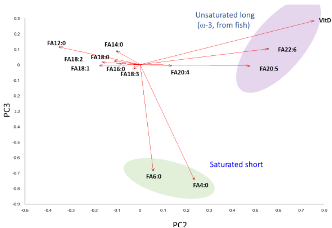
Fig.4.10 Result of free fatty acid dataset (PCA)
