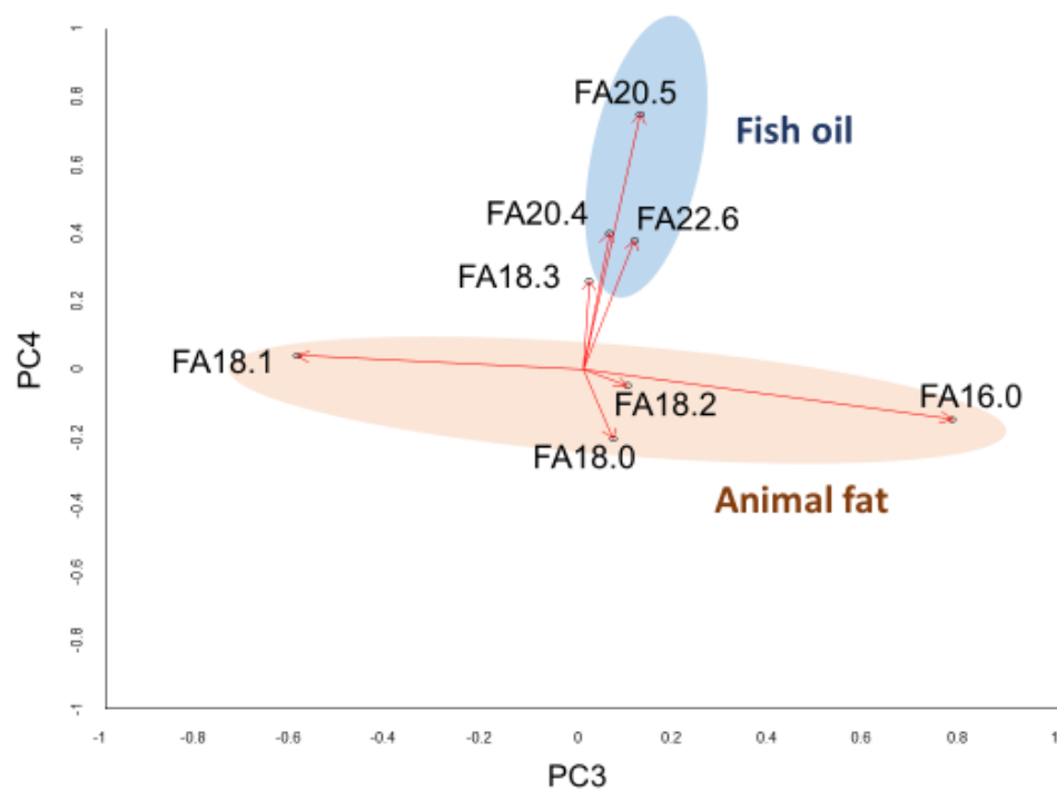
Fig.4.18 Result of fatty acid dataset (CPCA)
