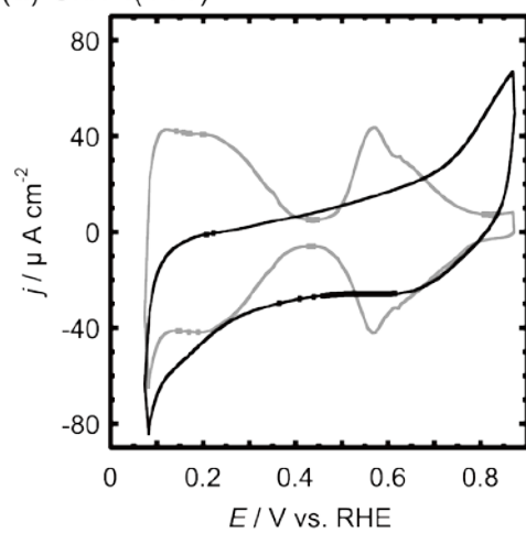
(b) Sn/Pt(100)
