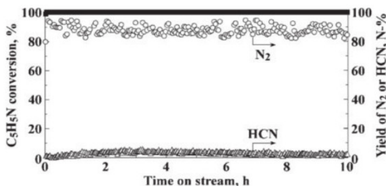
図 500°Cでのピリジン分解に対する褐鉄鉱の触媒性能
