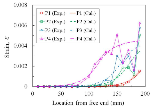
(d) Savoia et al.'s model
