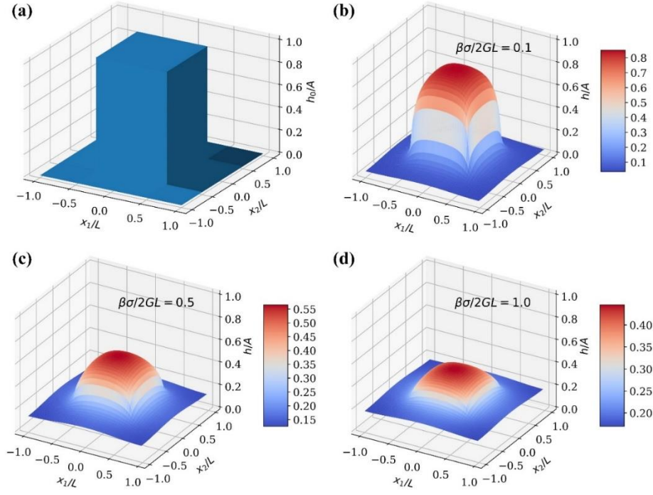
Fig. 3. (a) Initial profile; (b) \beta\sigma / 2GL = 0.1 ; (c) \beta\sigma / 2GL = 0.5 ; (d) \beta\sigma / 2GL = 1 .
