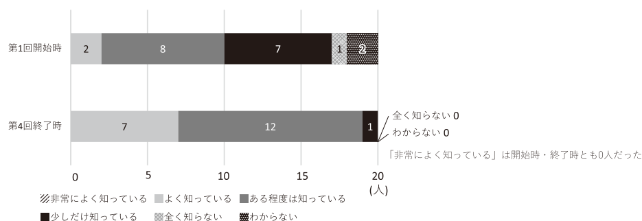
図 5-8 気候変動についての知識
