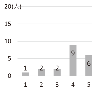
図 3-1-30 地域冷暖房
