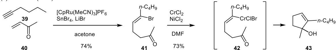
Scheme 1-6.
