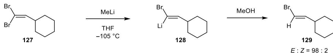
Scheme 3-4.
