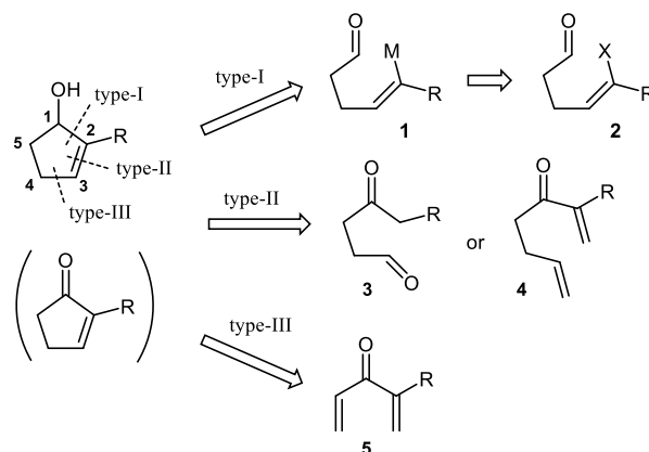
Scheme 1-2.
