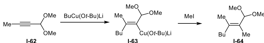
Scheme I-8.
