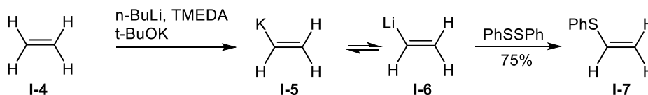
Scheme I-1.
