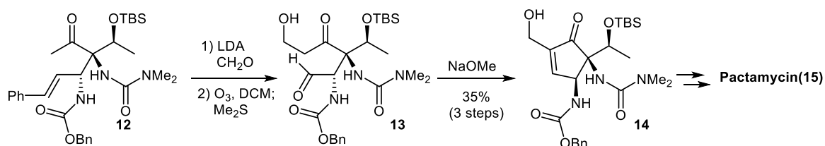
Scheme 1-3.
