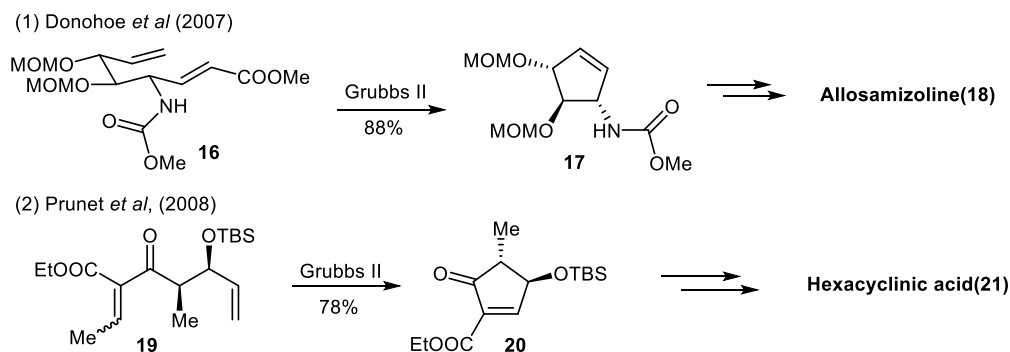
Scheme 1-4.
