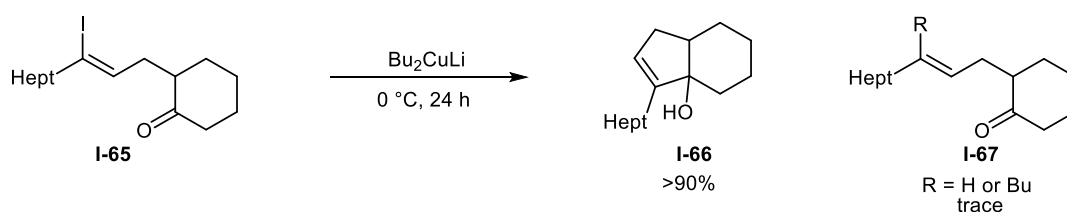
Scheme I-9.
