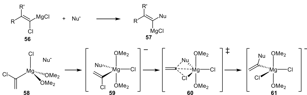
Scheme 1-9.
