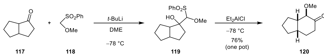
Scheme 2-8.
