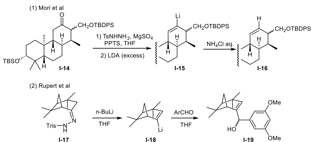
Scheme I-3.
