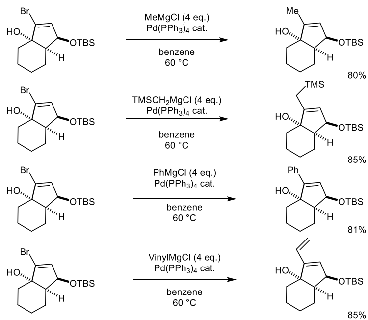
Scheme 3-8.
