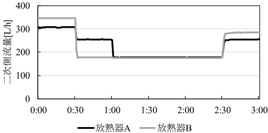
図 4-2 二次側流量
