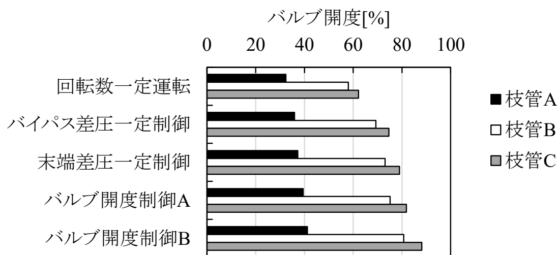
図 6-9 電動バルブの開度の平均値
