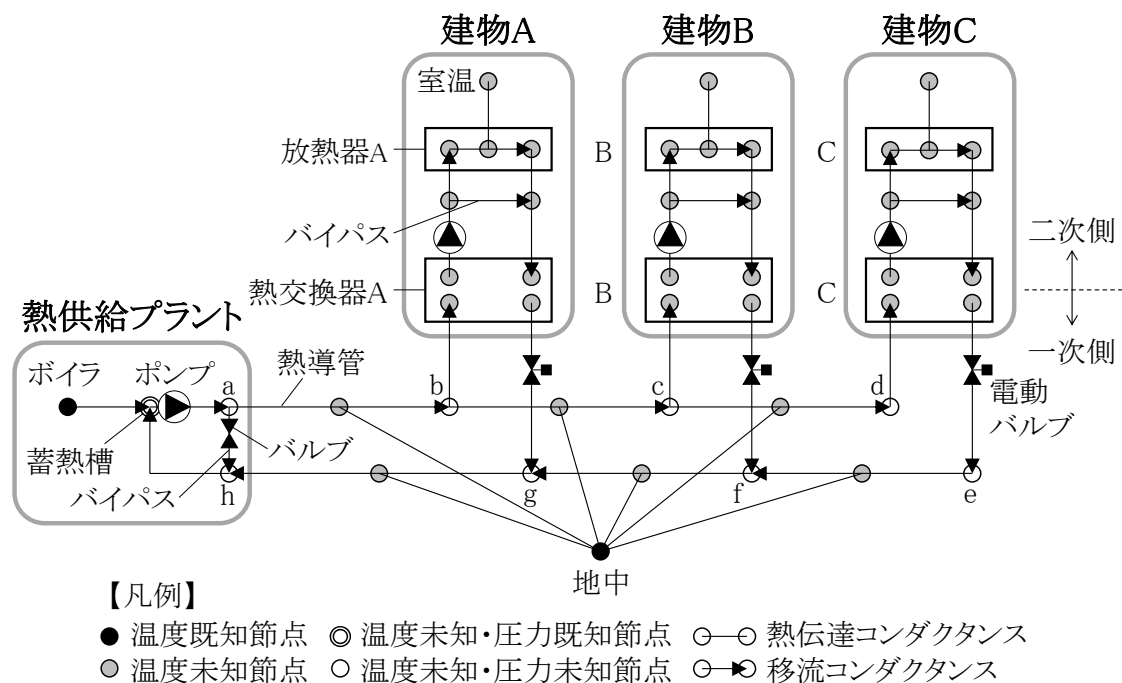
図 6-2 解析モデル
