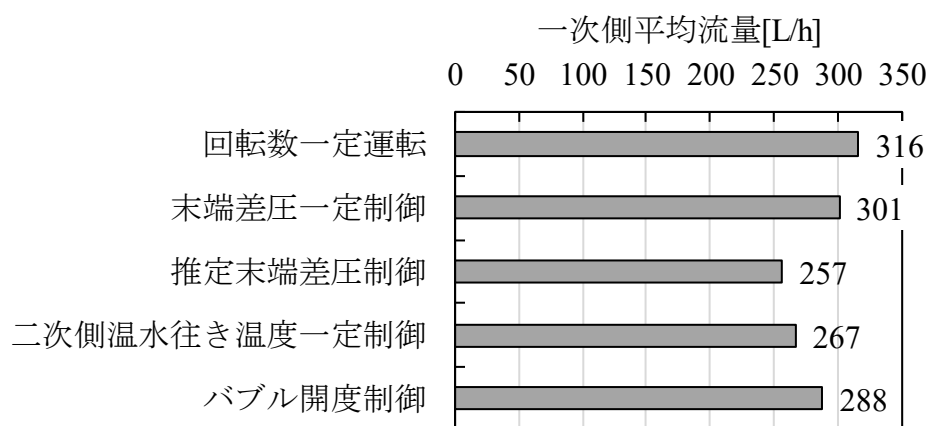
図 4-12 一次側平均流量
