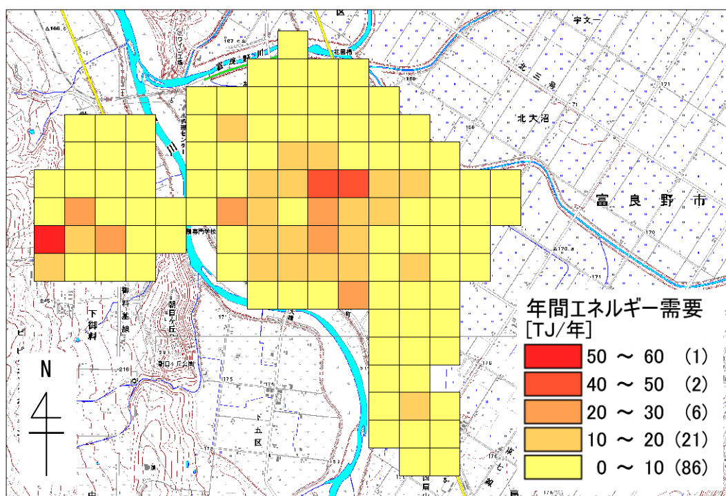
図3-6 年間エネルギー需要 注2)
