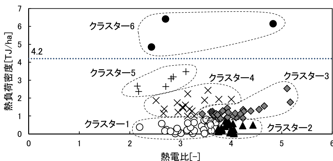
図 2-10 各クラスターの熱負荷密度と熱電比の関係
