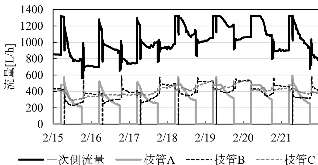
図 6-4 一次側流量
