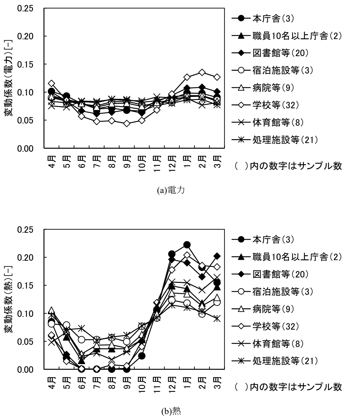
図 2-8 用途別の変動係数
