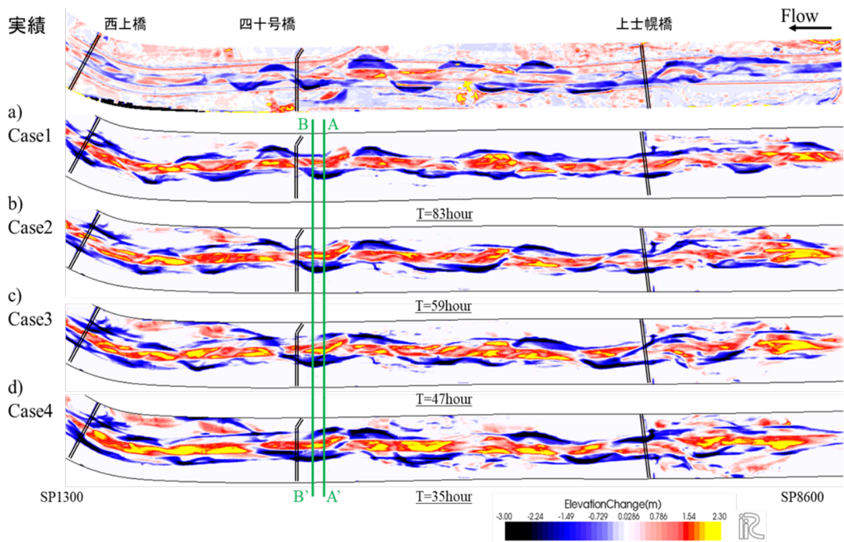
図4-11 積算流量が同じとなる時刻(図4-10の黒点)の河床変動量コンター図
