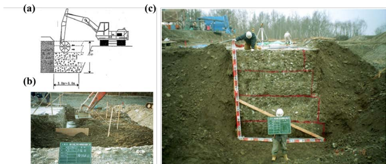
図6-5 十勝川水系札内川(KP12.6 右岸)における現地材料を活用したコンクリートウォールを用いた堤防基盤部分の侵食防護対策の試験工事
