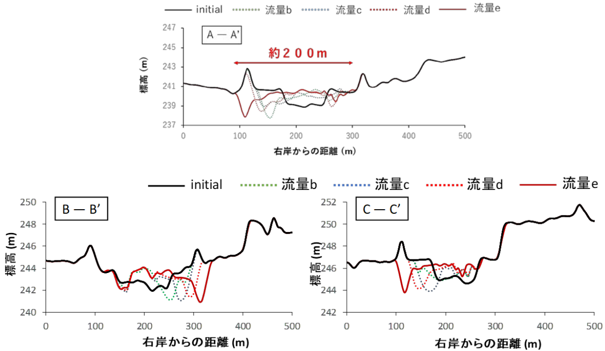
図 3-18 数値解析による堤防決壊箇所測線の横断形状の時間変化
