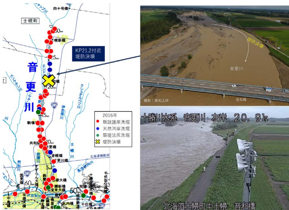
図 2-12 2016 年 8 月洪水による河岸侵食（侵食幅 20m 以上）の発生箇所（開発局提供 28) ）
