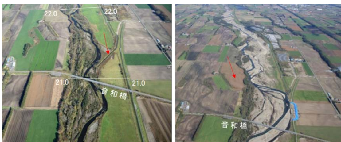
図 2-13 2016 年 8 月洪水前後の破堤地点 (KP21.2) の様子（開発局提供）
