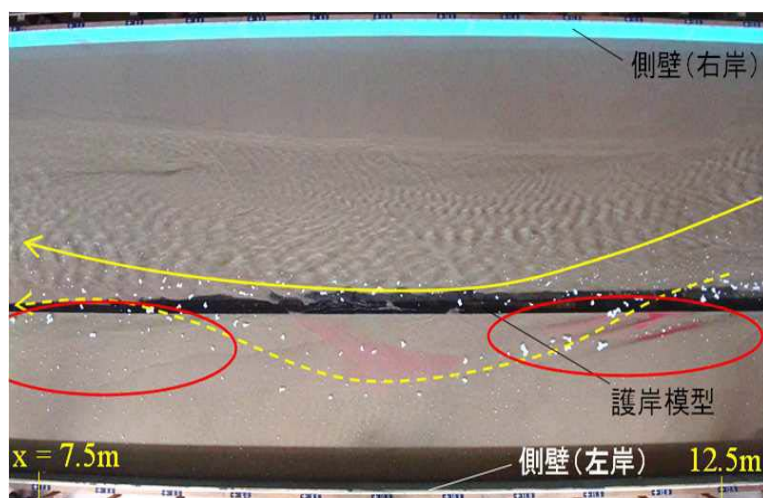
図 5-13 最大流量時の流況 (Run 3)
