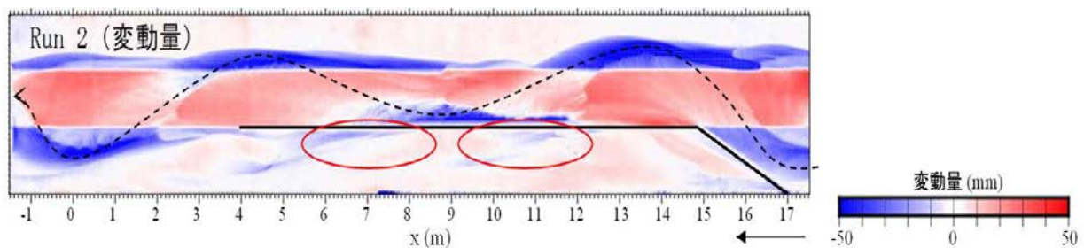
図 5-11 Run 2 の護岸模型周辺の河床変動量 （点線：主流位置，赤丸は護岸背後の洗掘箇所）
