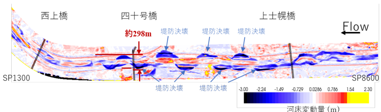
図 3-6 河床変動量コンター図
