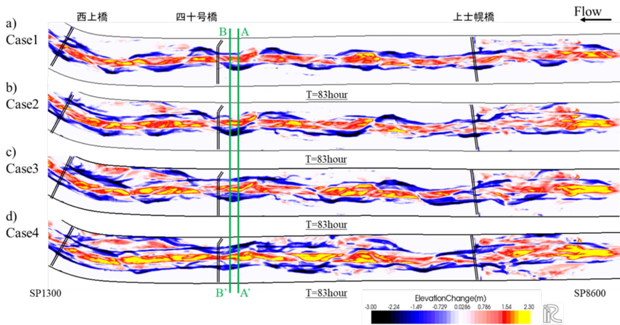
図 4-13 計算終了時の河床変動量コンター図
