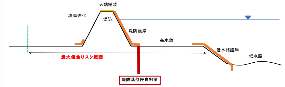
図6-4 施設対応による短期・中期的な対策案
