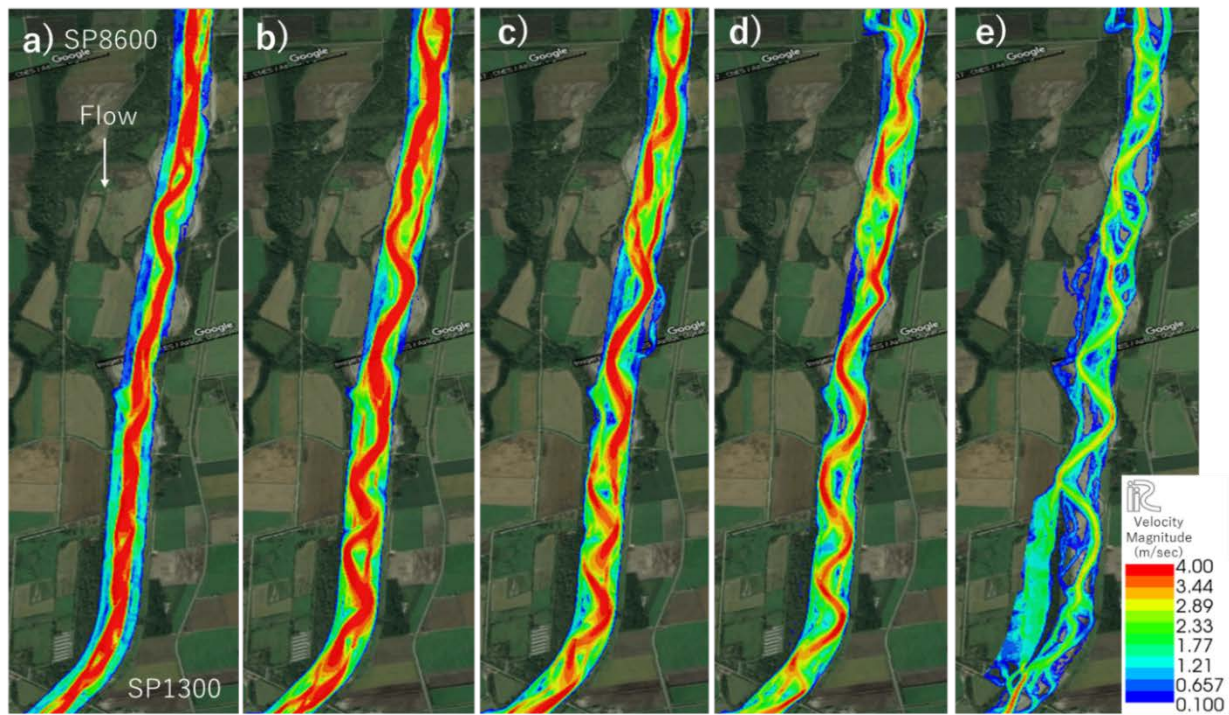
図 3-16 数値解析による流速(m/sec)の時間変化コンター図(画像背景: Google Earth 2016/9)
