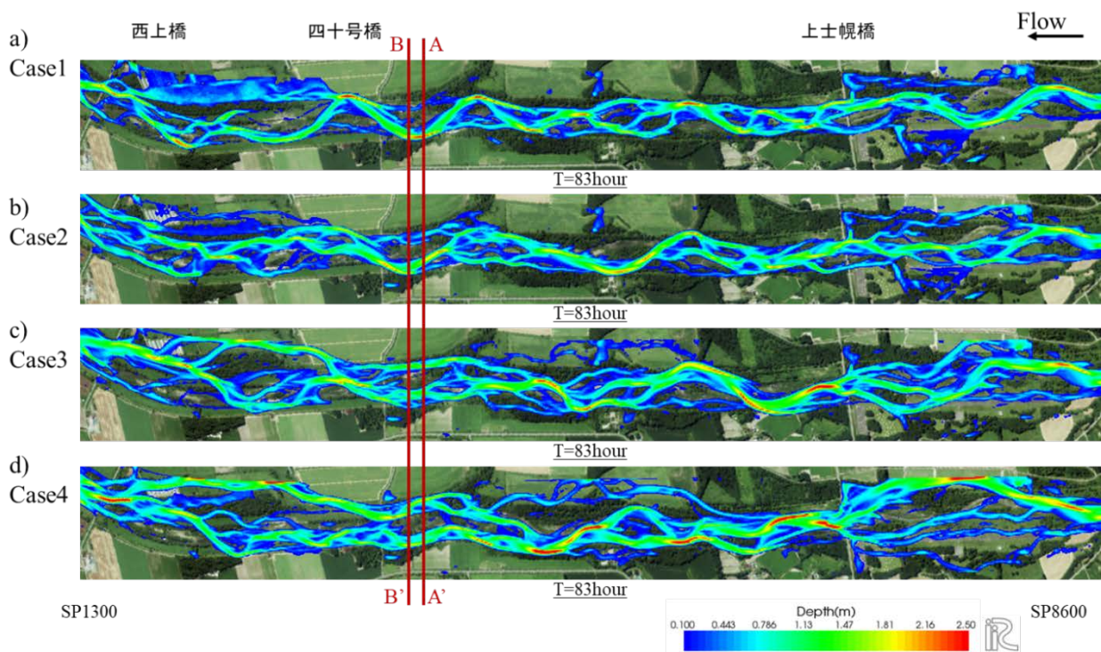
図 4-14 計算終了時(T=83 hour)の水深コンター図
