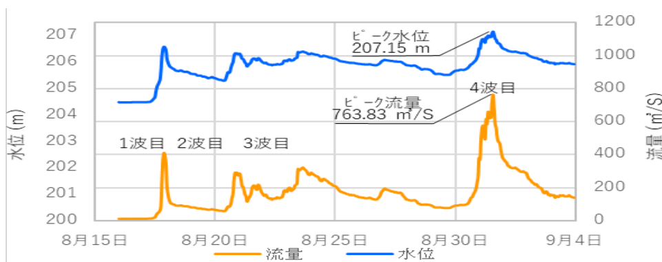
図 2-11 2016 年 8 月降雨前後における音更川(士幌観測所)の水位・流量ハイドログラフ(北海道開発局提供, 暫定値)
