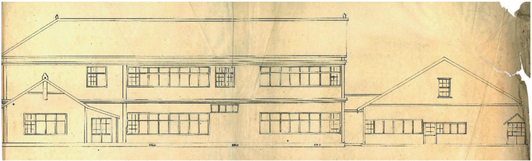
遠友夜学校校舎増築工事側面図(1928年頃)
