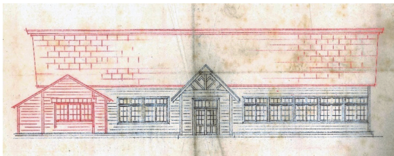
遠友夜学校旧校舎の正面図(1928年頃)
