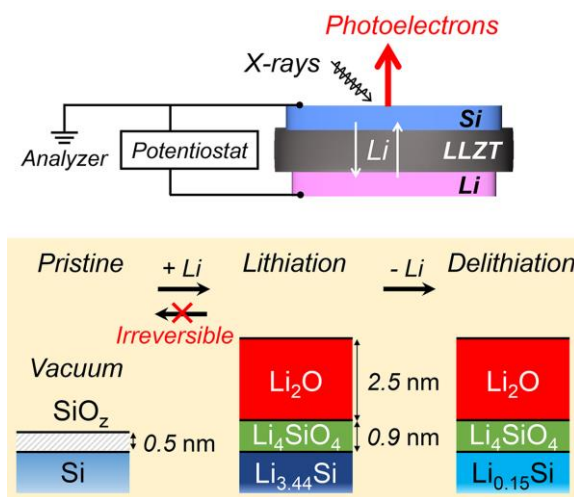
Figure 1. その場 XPS 法によって観測された Si 薄膜負極の初回 Li 挿入・脱離反応による変化
