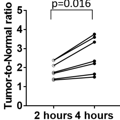
D. GBM
