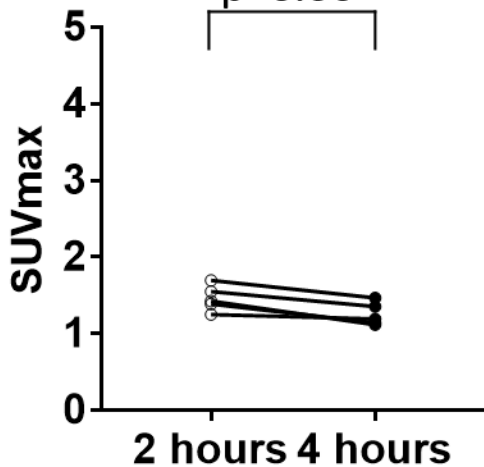
A. non-GBM
