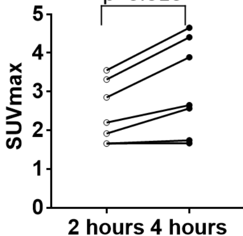
B. GBM
