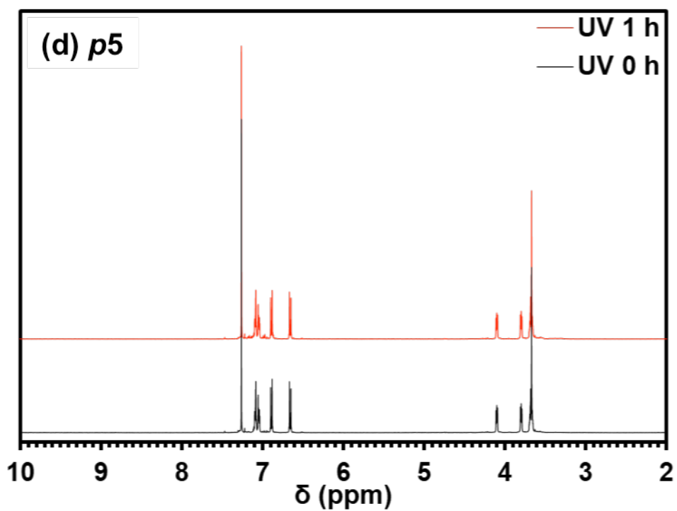
Figure 10 (continued). ^1\text{H} NMR spectra of (c) p4 and (d) p5 upon photoirradiation.
