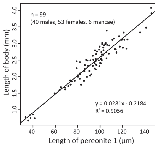
図2. 第1胸節長と体長の関係 (雄40個体, 雌53個体, 幼体6個体の結果に基づく).
