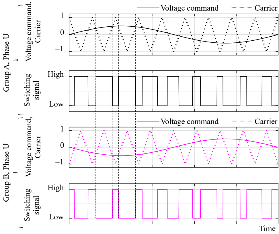
図 5.2 従来の逆位相スイッチングによる PWM の概要
