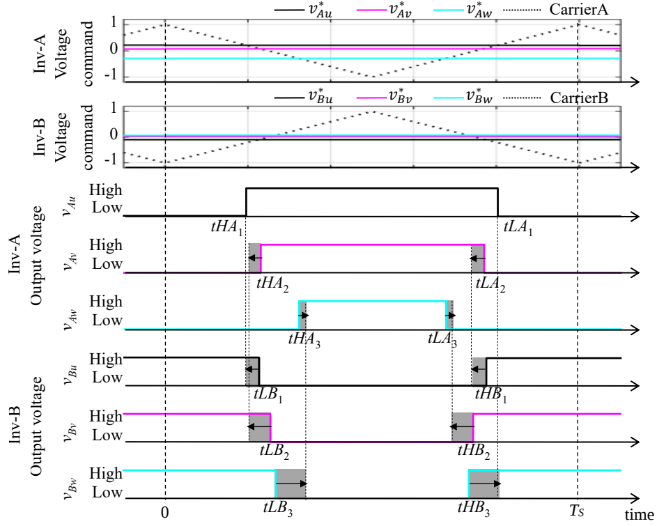
図 4.2 提案するスイッチング制御の概要
