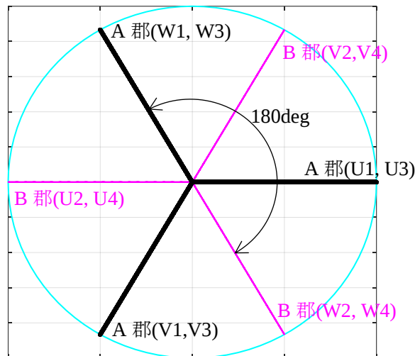
図 5.12 巻線の位相関係 (位相差 180 deg)
