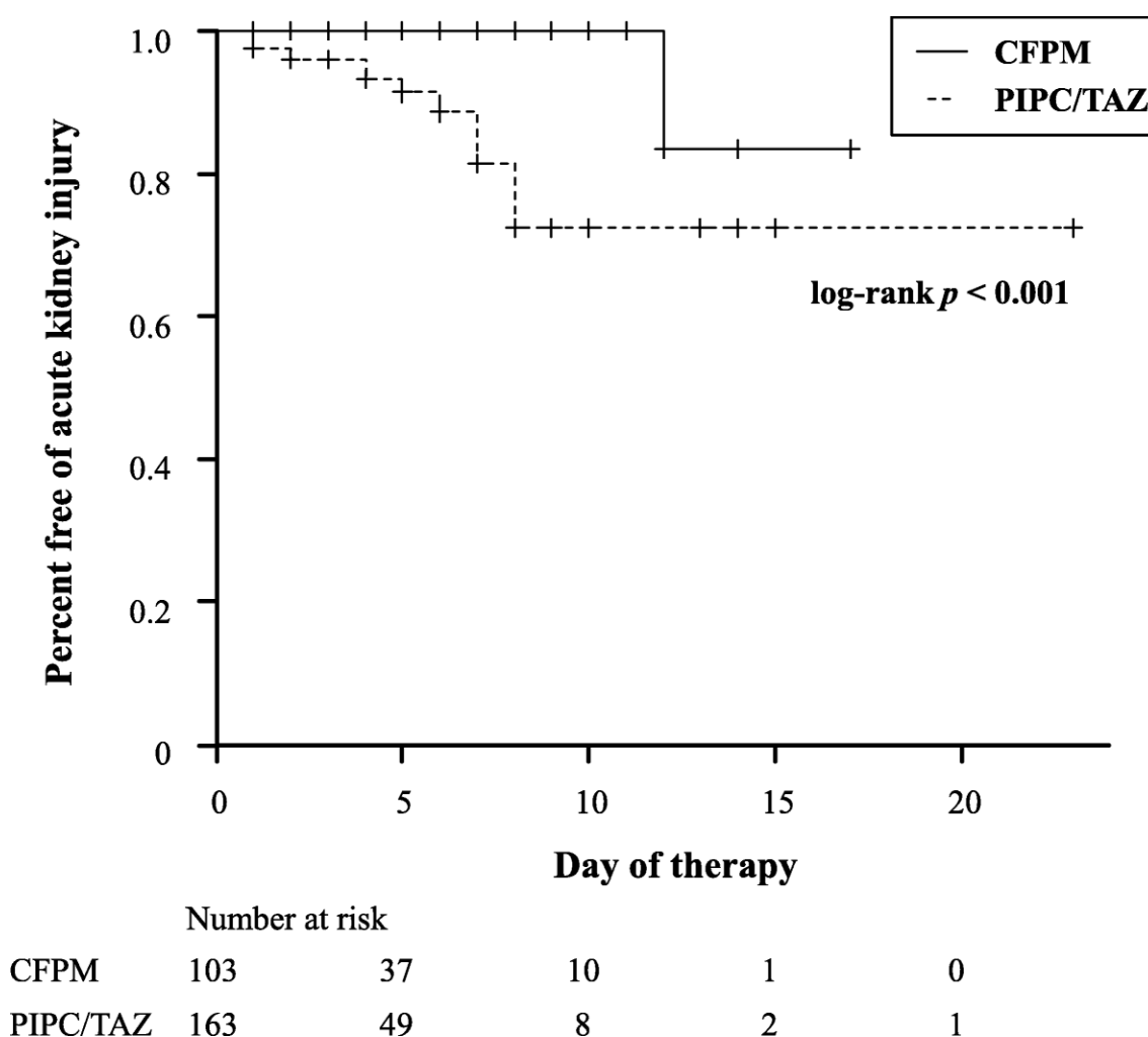
Figure 2 PIPC/TAZ および CFPM の急性腎障害発症の Kaplan-Meier 曲線
