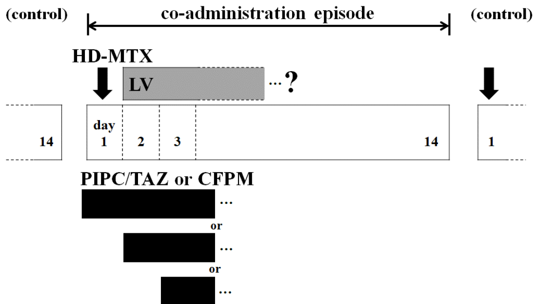
Figure 6 HD-MTX 施行患者における PIPC/TAZ および CFPM の相互作用研究のシェーマ
