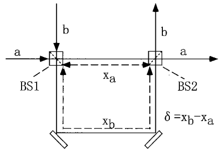
図2 マッハツェンダー干渉計 Fig.2 Analysis of a Mach-Zehnder interferometer.
