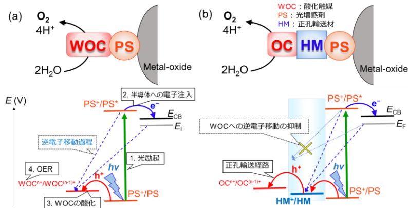
Fig. 1 (a) 触媒-光増感剤連結型光酸素発生電極および (b) 正孔輸送部位導入型光酸素発生電極の概略図
