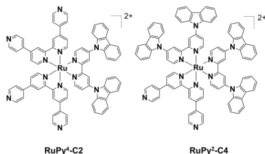
Fig. 4 ピリジル基・cbz 基導入型 Ru(II) 色素
