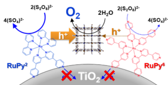
Fig. 3 光増感ナノ粒子 RuPy n @TiO 2 を用いた光化学的 OER。
