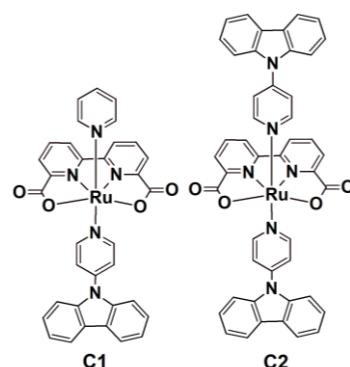
Fig. 2 cbz 修飾型 OER 触媒 C1 および C2 。
