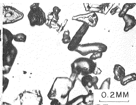
Photo. 10. 1/cc 0805 19 Dec., 1960.
