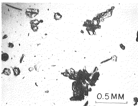
Photo. 9. 1.8/cc 2205 18 Dec., 1960.
