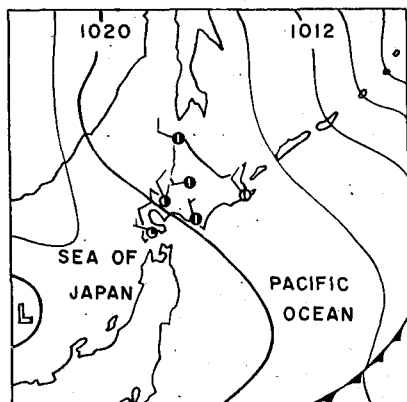
Fig. 4. 0900 20 Dec., 1960.
