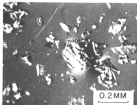
Photo. 11. 2.4/cc 1436 20 Dec., 1960.
