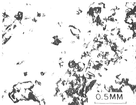
Photo. 7. 1.4/cc 2213 17 Dec., 1960.
