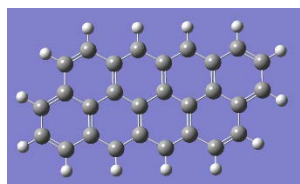
Peri-naphthacenonaphthacene
