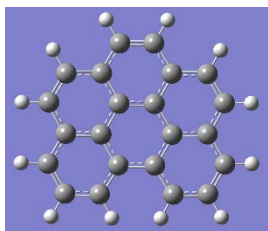
1,12-Benzoperylene
