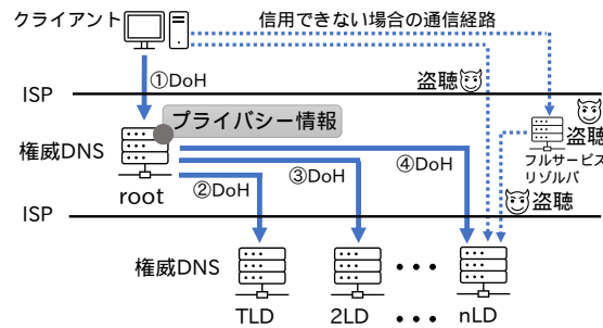
図2 提案手法の構成
