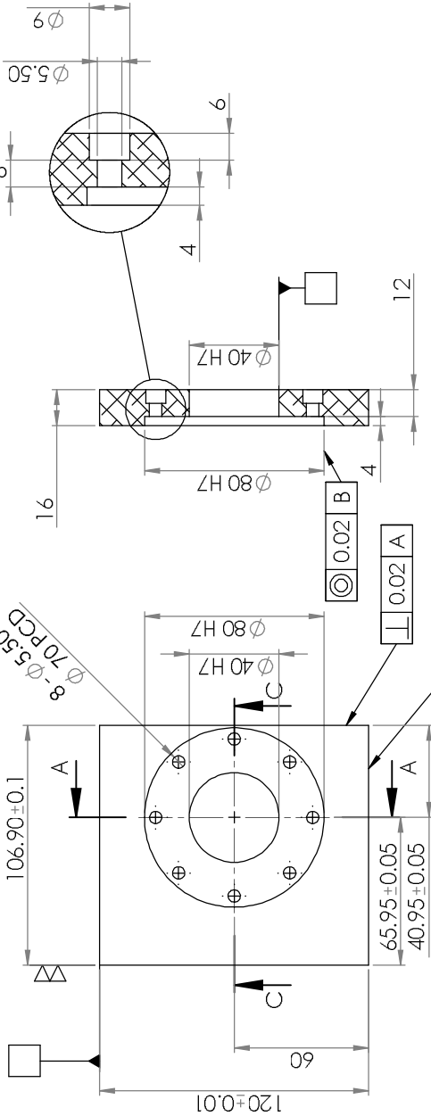
SECTION A-A SCALE 1 : 2
