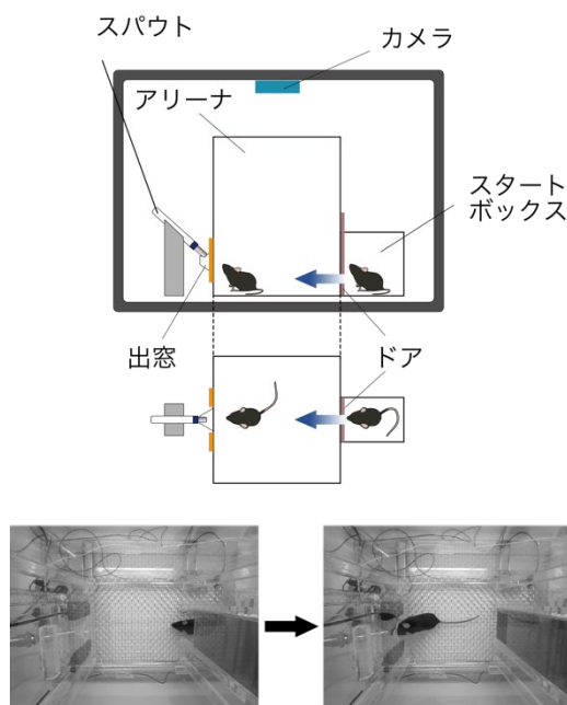
図 14. 微細行動分析システム
