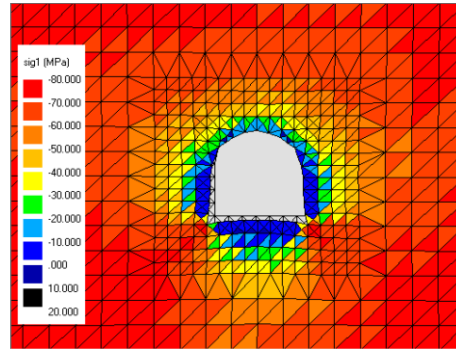
(d) Just before rockburst
