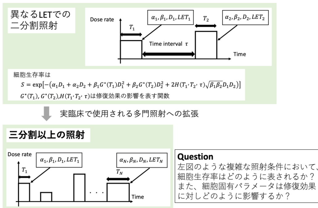
図 1.8 第一段階の研究の概要。先行研究(Zaider and Rossi, 1980)で想定された二分割照射の模式図とその細胞生存率の式に加え、この研究で検討した三分割以上の照射での線量率構造を示した。
