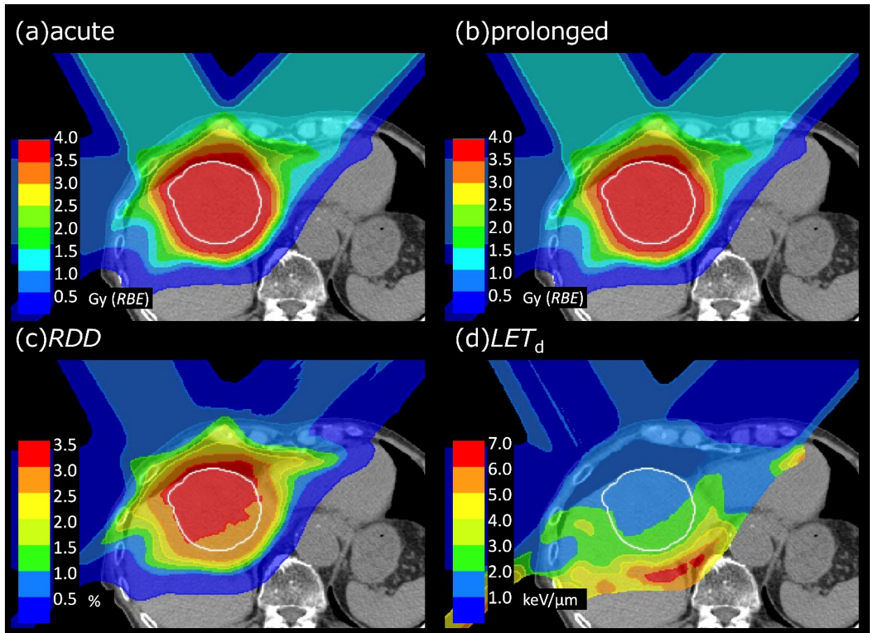
図 3.8 肝臓がんのケースにおける線量と LET_d 分布。(a)瞬間照射における生物線量。(b) (\alpha/\beta)_x = 14.3 Gy, T_{1/2} = 32.4 min に設定した場合の、時間がかかった照射における生物線量分布。総照射時間は 29 min とした。(c) (a)と(b)から計算された RDD 分布。(d)このプランにおける LET_d 分布。CTV の輪郭を画像の中心に白線で示した。
