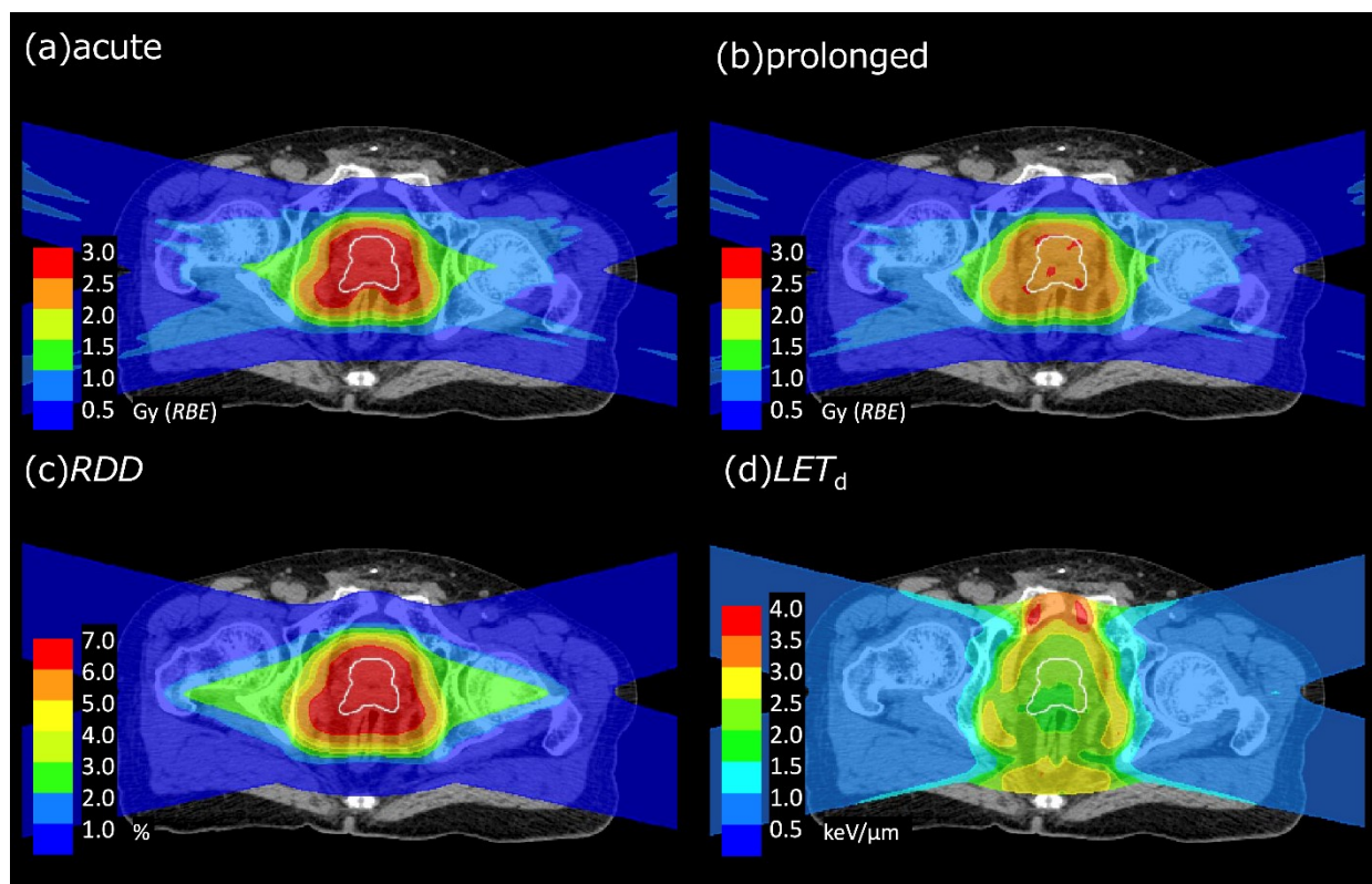
図 3.7 前立腺がんのケースにおける線量と LET_d 分布。(a)瞬間照射における生物線量。(b) (\alpha/\beta)_x = 1.49 Gy, T_{1/2} = 32.4 min に設定した場合の、時間がかかった照射における生物線量分布。総照射時間は 31 min とした。(c) (a)と(b)から計算された RDD 分布。(d)このプランにおける LET_d 分布。CTV の輪郭を画像の中心に白線で示した。
