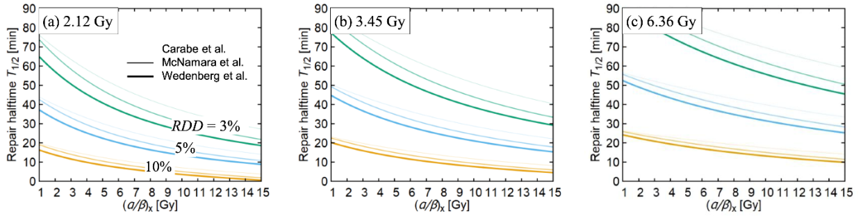
図 3.11 SOBP center における 30 min の continuous irradiation において、三種類の RBE モデルから得られた、RDD の等高線。各曲線に対応する RDD の値は図 3.11(a)に示している。
