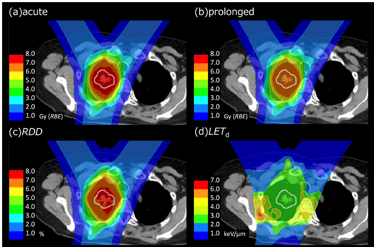
図 3.6 肺がんのケースにおける線量と LET_d 分布。(a)瞬間照射における生物線量。(b) (\alpha/\beta)_x = 3.9 \text{ Gy} , T_{1/2} = 32.4 \text{ min} に設定した場合の、時間がかかった照射における生物線量分布。総照射時間は 29 min とした。(c) (a)と(b)から計算された RDD 分布。(d)このプランにおける LET_d 分布。CTV の輪郭を画像の中心に白線で示した。
