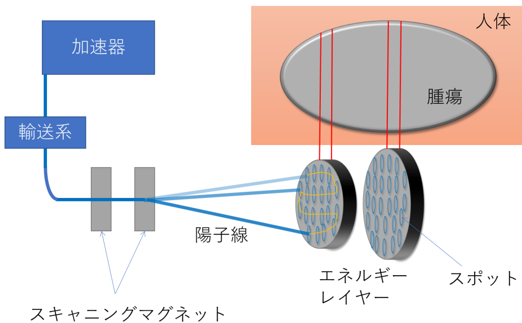
図 1.7 スキャニング照射法の一つである、スポットスキャニング照射の模式図。ビーム輸送の詳細や陽子線照射ノズルの構造は簡略化して描述した。また、エネルギーレイヤーについては部分的に抜き出して表示した。
