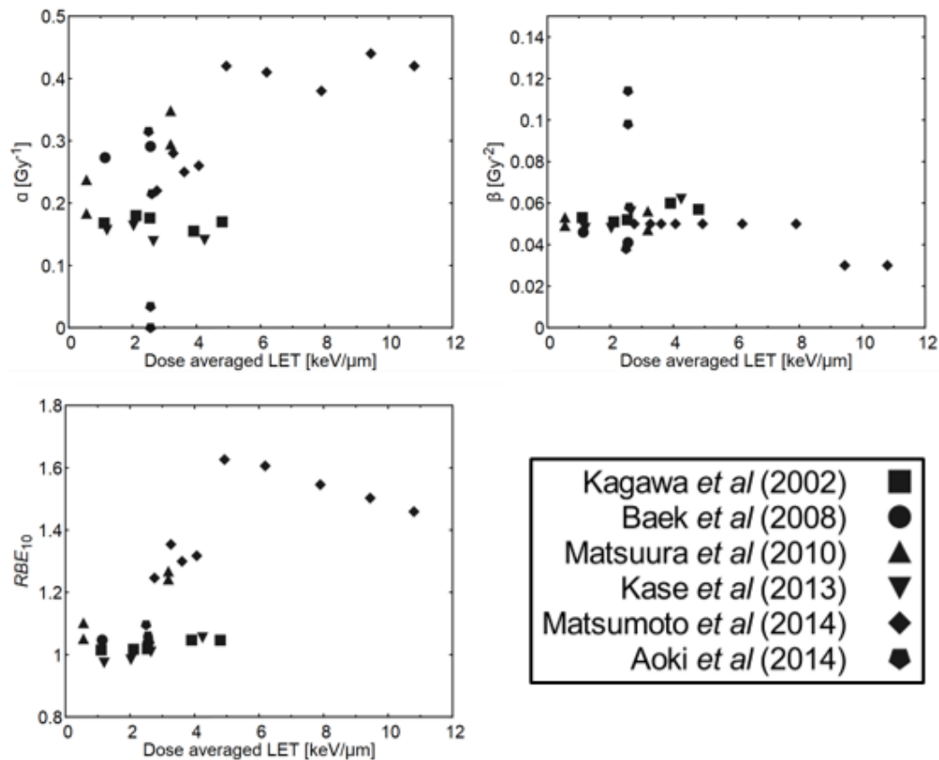
図 2.3 Paganetti がまとめた、HSG 細胞に対する陽子線照射で得られた LQ パラメータと RBE_{10} (Paganetti, 2014b) を、横軸を LET_d にとってプロットした図。元論文 (Aoki-Nakano et al., 2014; Baek et al., 2008; Kagawa et al., 2002; Kase et al., 2013; Matsumoto et al., 2014; Matsuura et al., 2010) が載せていない LET_d については Paganetti によって Janni の参照表 (Janni, 1982) からの取得、またはシミュレーションが行われ、LQ パラメータおよび LET が得られている。
