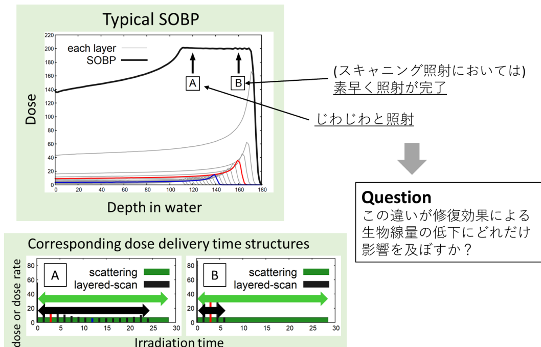
図 1.9 第二段階の研究の概要。スキャニング照射法における典型的な SOBP について、SOBP 内の異なる二つの深さの位置における線量率構造を示した図。散乱体法で想定される、定線量率での照射における線量率構造についても同時に示している。
