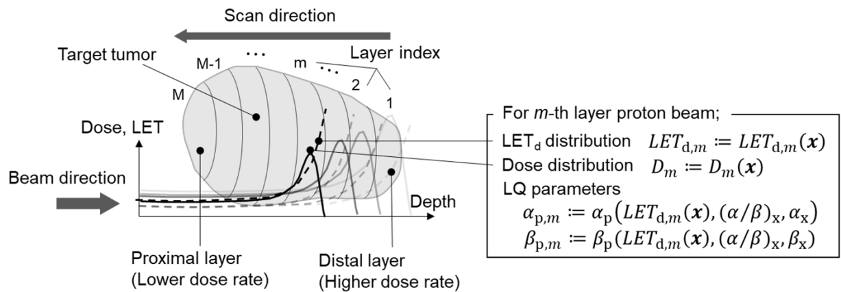
図 4.1 レイヤースキャン型陽子線照射法における典型的な線量付与構造の模式図と、生物モデルで用いたパラメータ。腫瘍は 1 から M までの複数のエネルギーレイヤーに分割され、それぞれのレイヤーに対応する線量・LET d (それぞれ実線と点線で表示)が順番に付与される。 m はレイヤーの index である。陽子線に対する LQ モデルにおける一次と二次の項( \alpha_p と \beta_p )は、LET d,m への依存性により、それぞれのレイヤースキャンごとに異なる値を取る。この依存性は本研究では McNamara の RBE モデルを使用して表現した(McNamara et al., 2015)。
