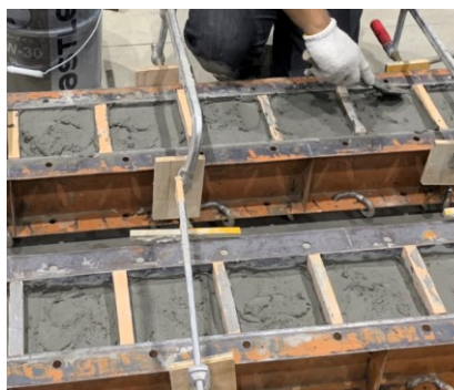
(d) Casting of PCM in two layers
