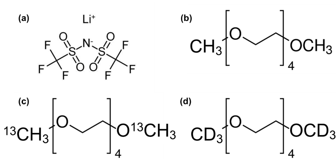
Figure 2-1. Molecule structure of (a) LiTFSI, (b) TEGDME, (c) ^{13}\text{CH}_3\text{-TEGDME} , and (d) \text{CD}_3\text{-TEGDME} .
