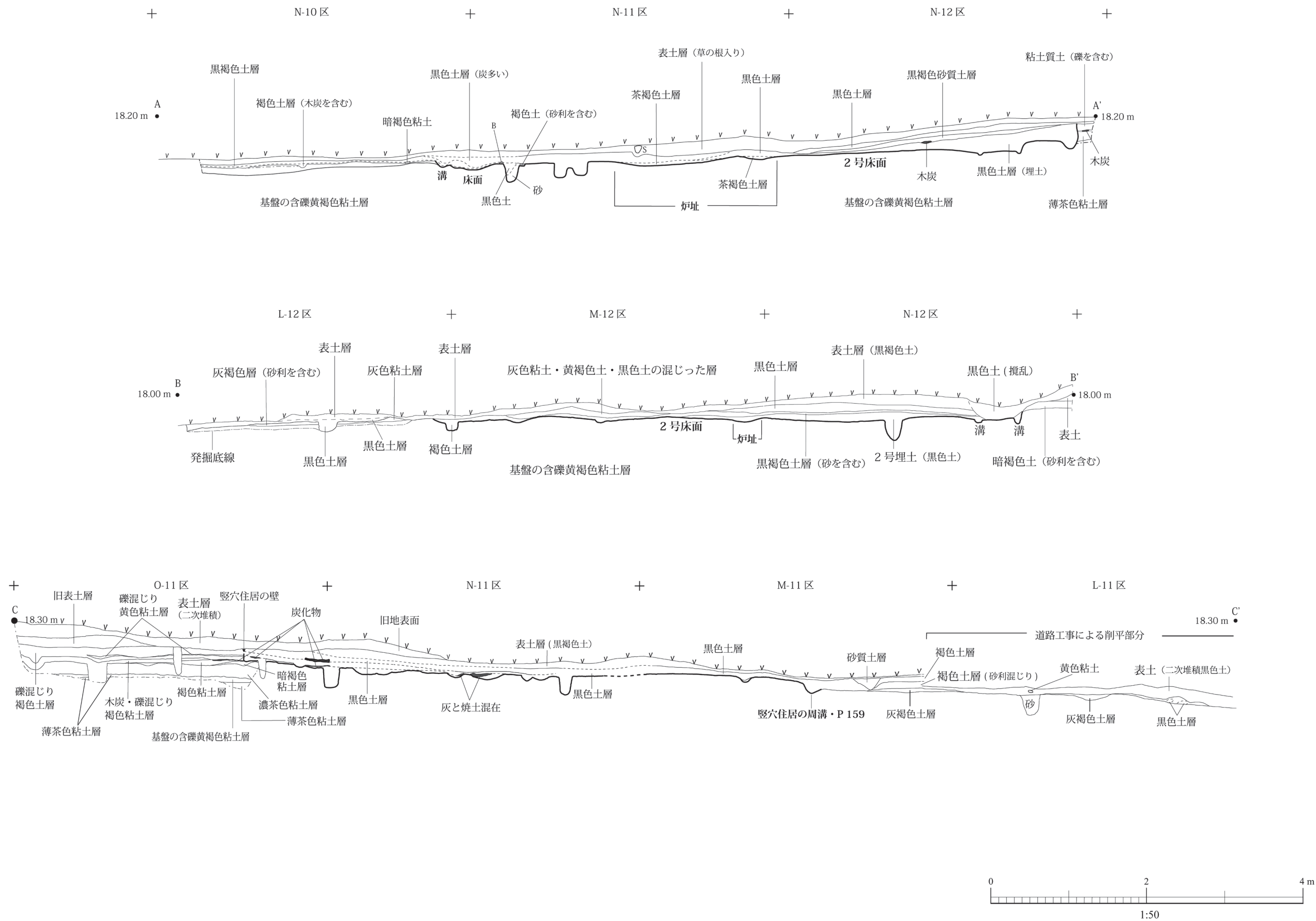
第 8 図 2 号竪穴住居址土層断面図 (1) A-A' (南北)・(2) B-B' (東西)・(3) C-C' (東西)
