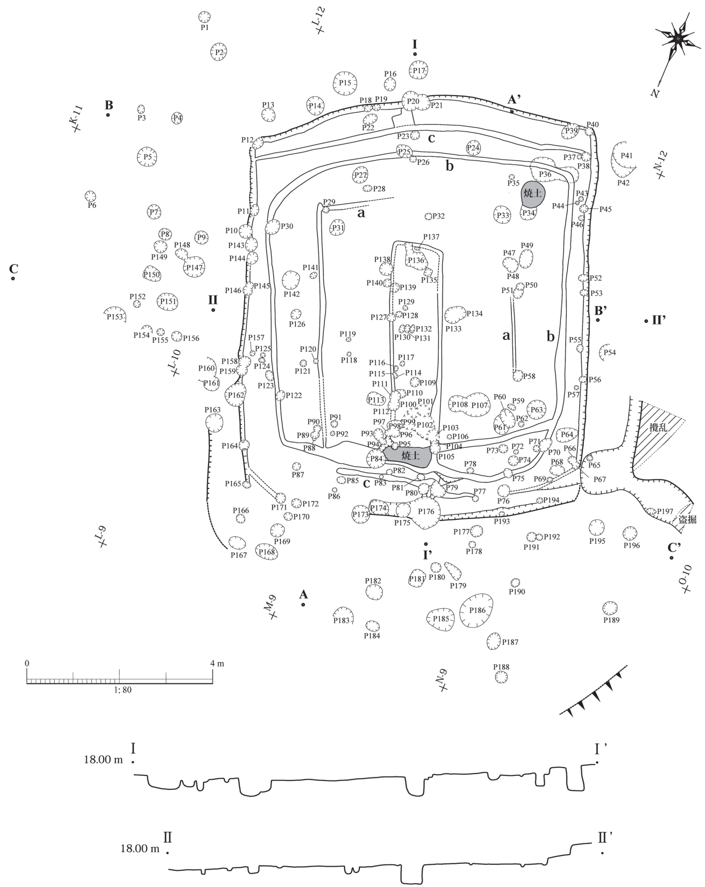
第7図 2号竖穴住居址平面図
