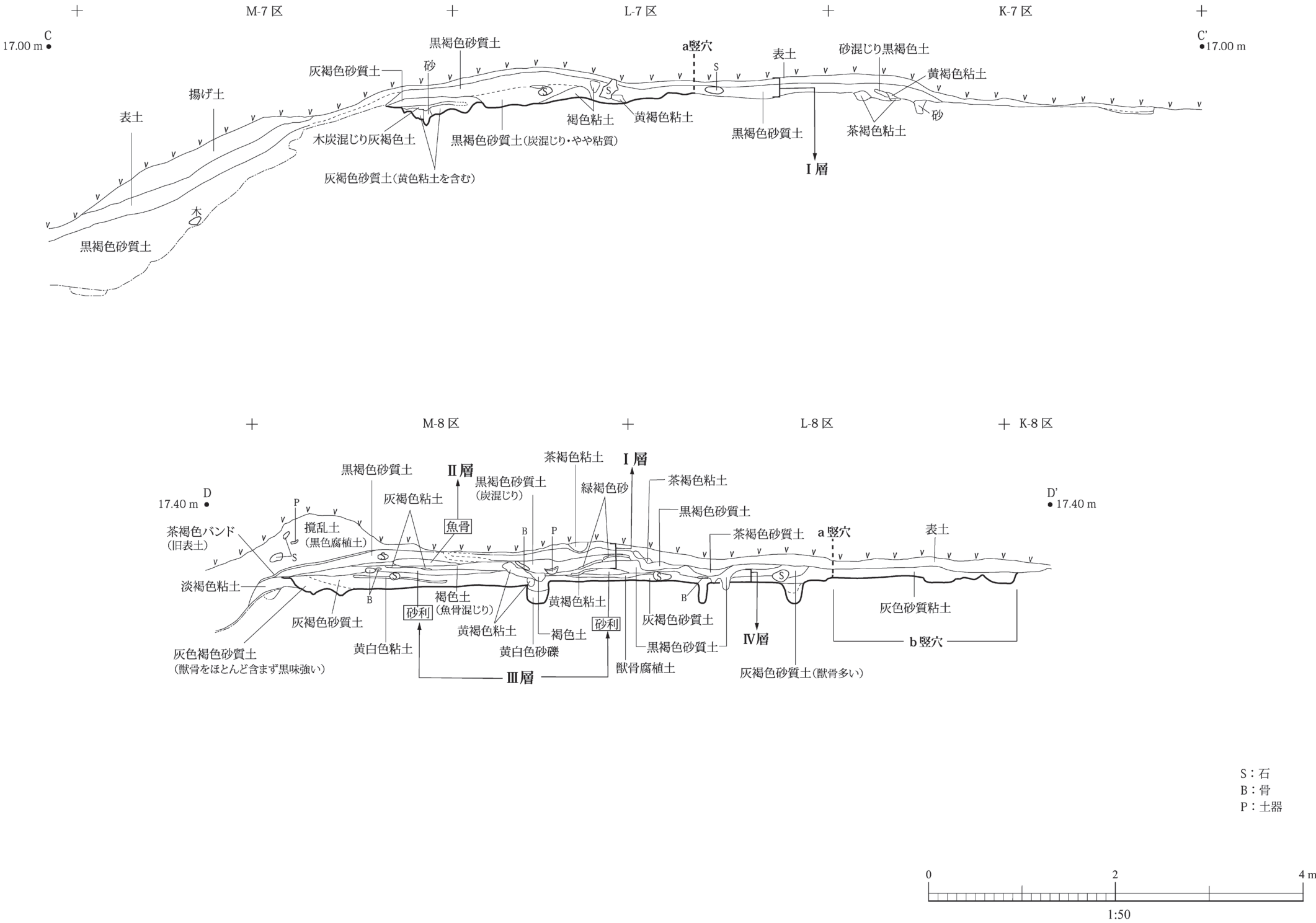
3 図 3号竪穴住居址土層断面図(2) C-C' (東西)・D-D' (東西)
